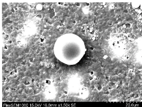
Obrázek 47- Zrna písku
