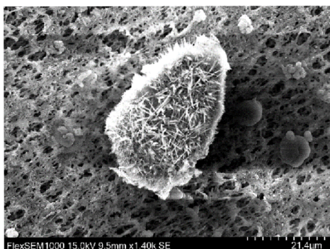
Obrázek 46- Krystaly vápníku
