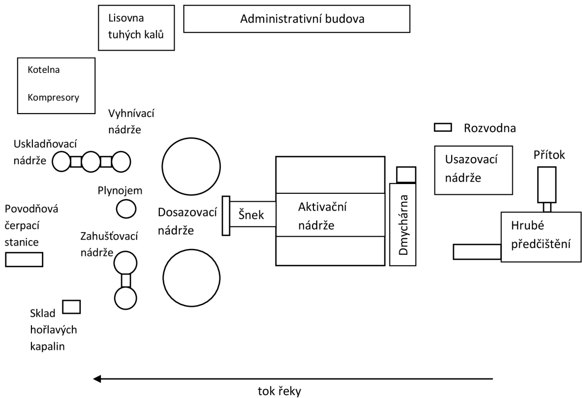
Obrázek 12- Schéma ČOV Havlíčkův Brod
