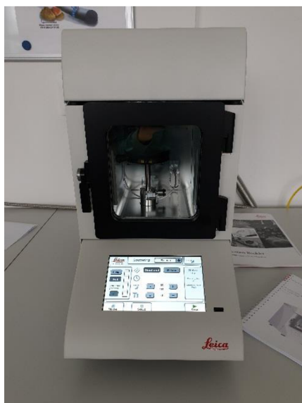
Obrázek 10- Nprašovač kovů a nprašené vzorky
