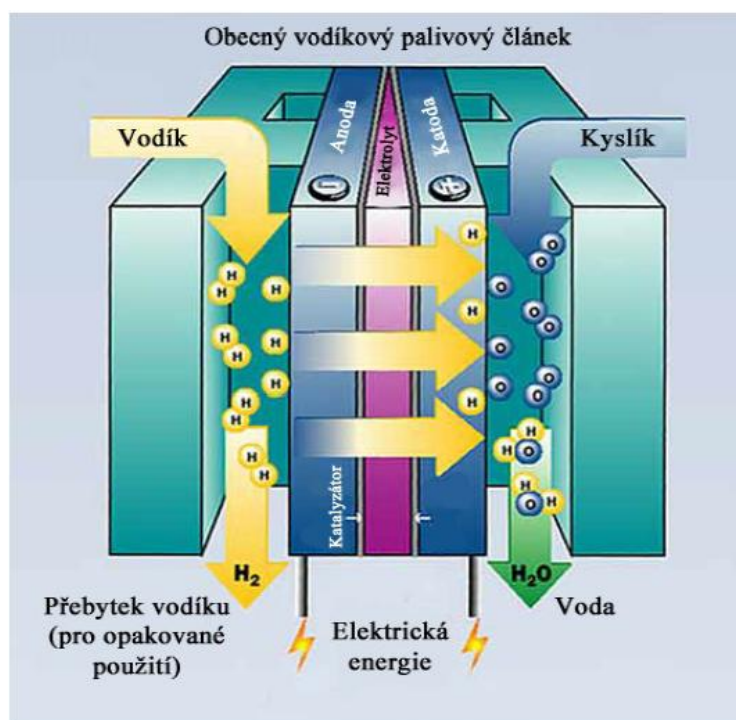
Obr. 1 Schéma palivového článku [5]
