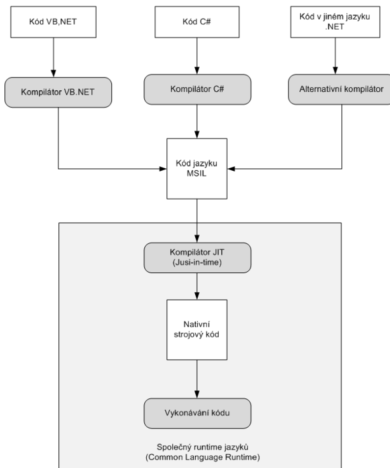
Obrázek 8.2: Kompilace webové stránky ASP.NET
