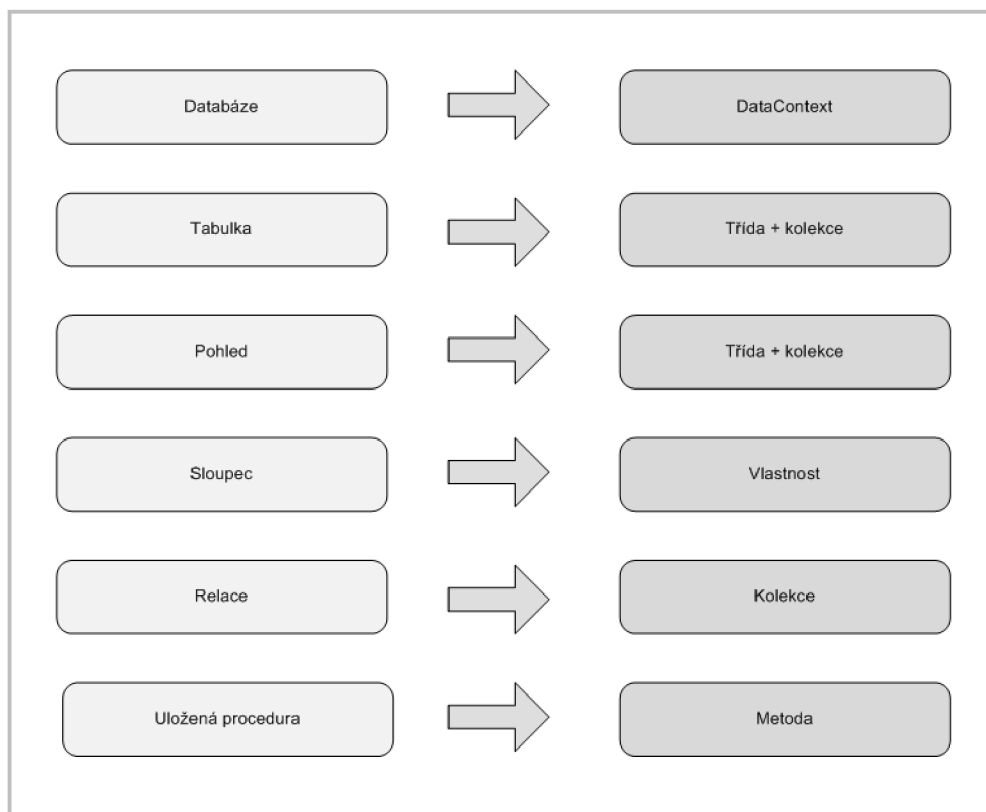
Obrázek 8.9: Diagram mapování LINQ to SQL
