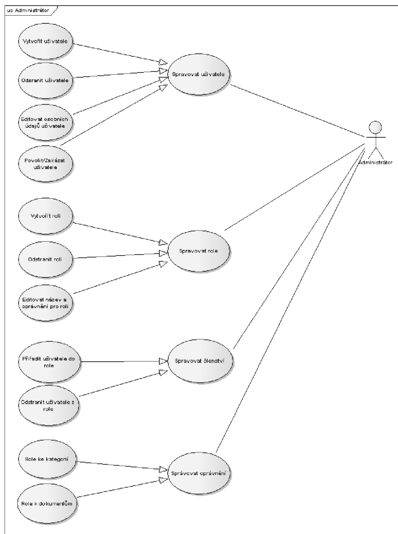
Obrázek 7.2: Use Case diagram - administrátor
