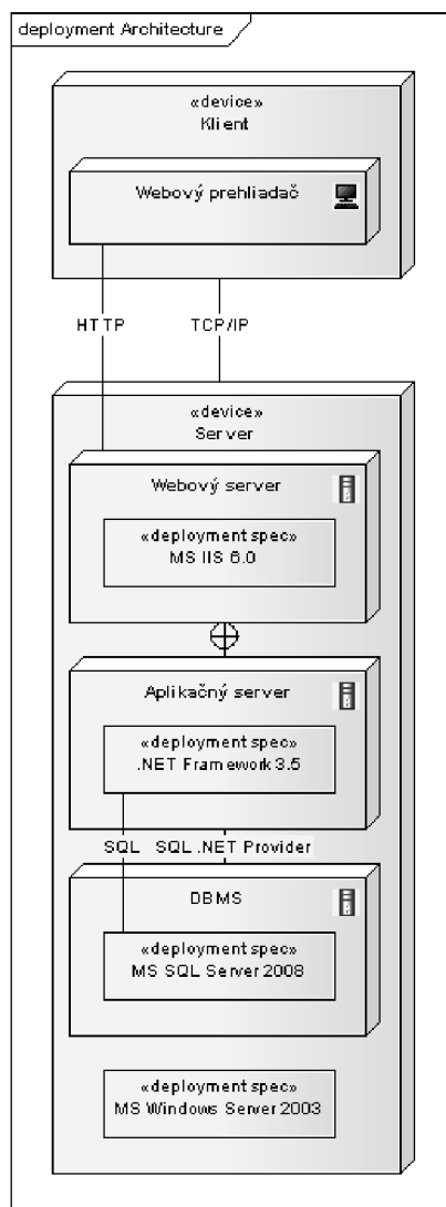
Obrázek 7.6: Architektura klient-server
