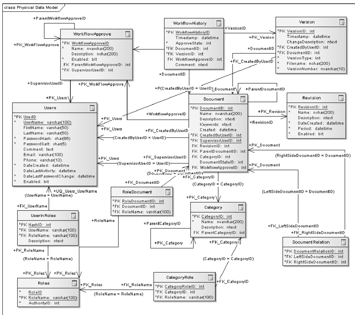
Obrázek 7.3: Entitně relační diagram
