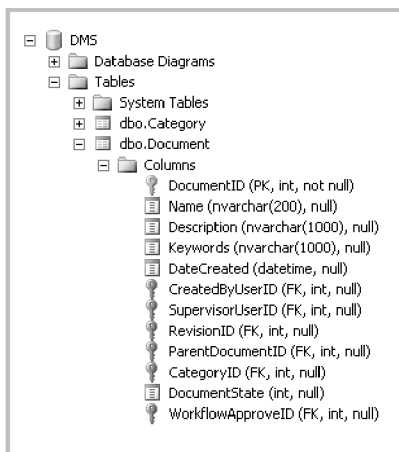
Obrázek 8.7: Tabulka Document s referencí na sebe sama (sloupec ParentDocumentID)
