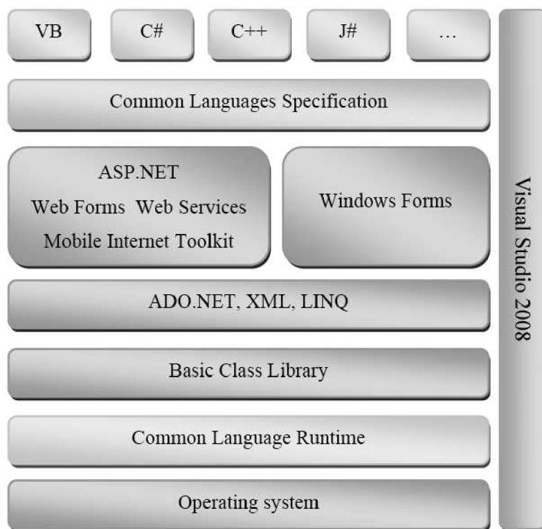
Obrázek 8.1: Diagram .NET Frameworku 3.5
