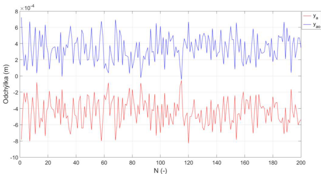
Obrázok 4.43 Odchýlky zväzku v priamom a spätnom kanáli pre model A sledujúci recipročné vlastnosti kanálu, kde y_a predstavuje odchylenie zväzku v priamom kanáli a y_{a_0} predstavuje odchylenie v spätnom kanáli
