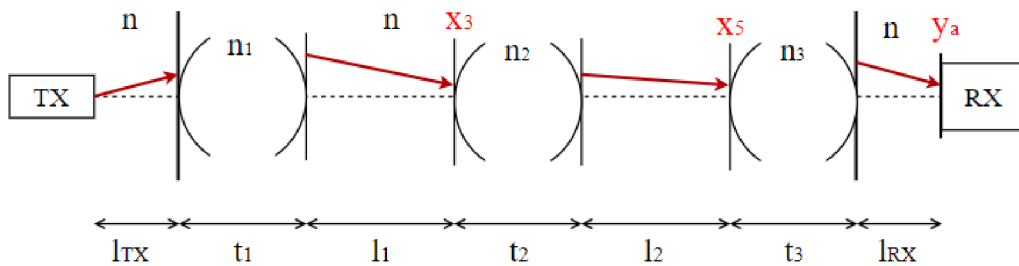
Obrázok 4.5 Model kaskádnej turbulencie pre modifikovanú metódu ETG
