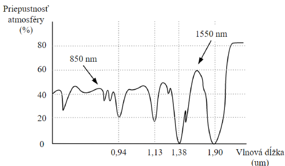
Obrázok 1.1 Spektrálna závislosť priepustnosti atmosféry [4]
