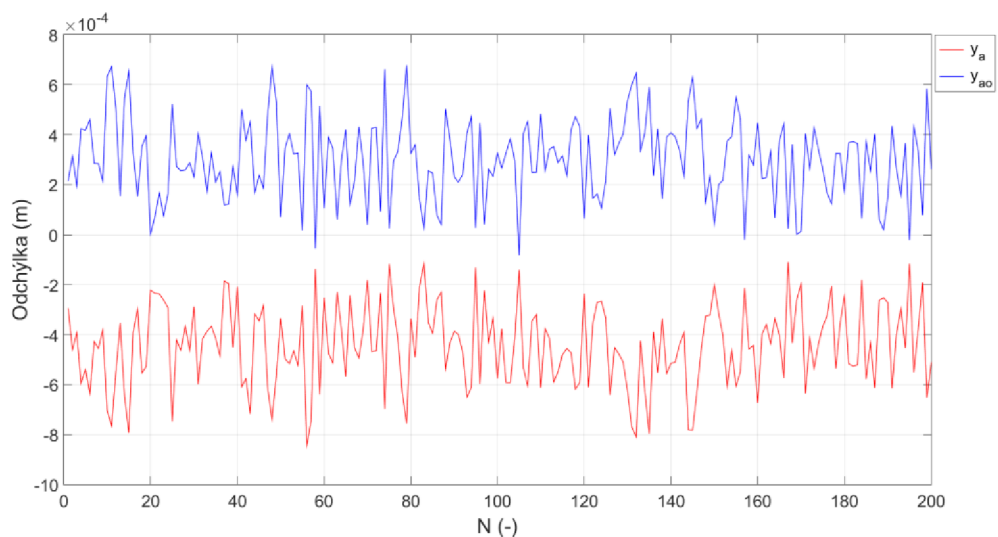
Obrázok 4.46 Odchýlky zväzku v priamom a spätom kanáli pre model B sledujúci recipročné vlastnosti kanálu
