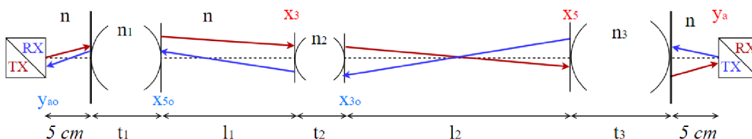
Obrázok 4.38 Náhodne generované turbulentné prostredie tvorené troma turbulentnými celami
