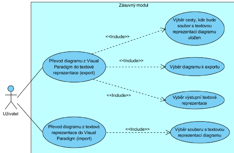
Obrázek 5.1: Diagram případů užití vyvíjeného zásuvného modulu
