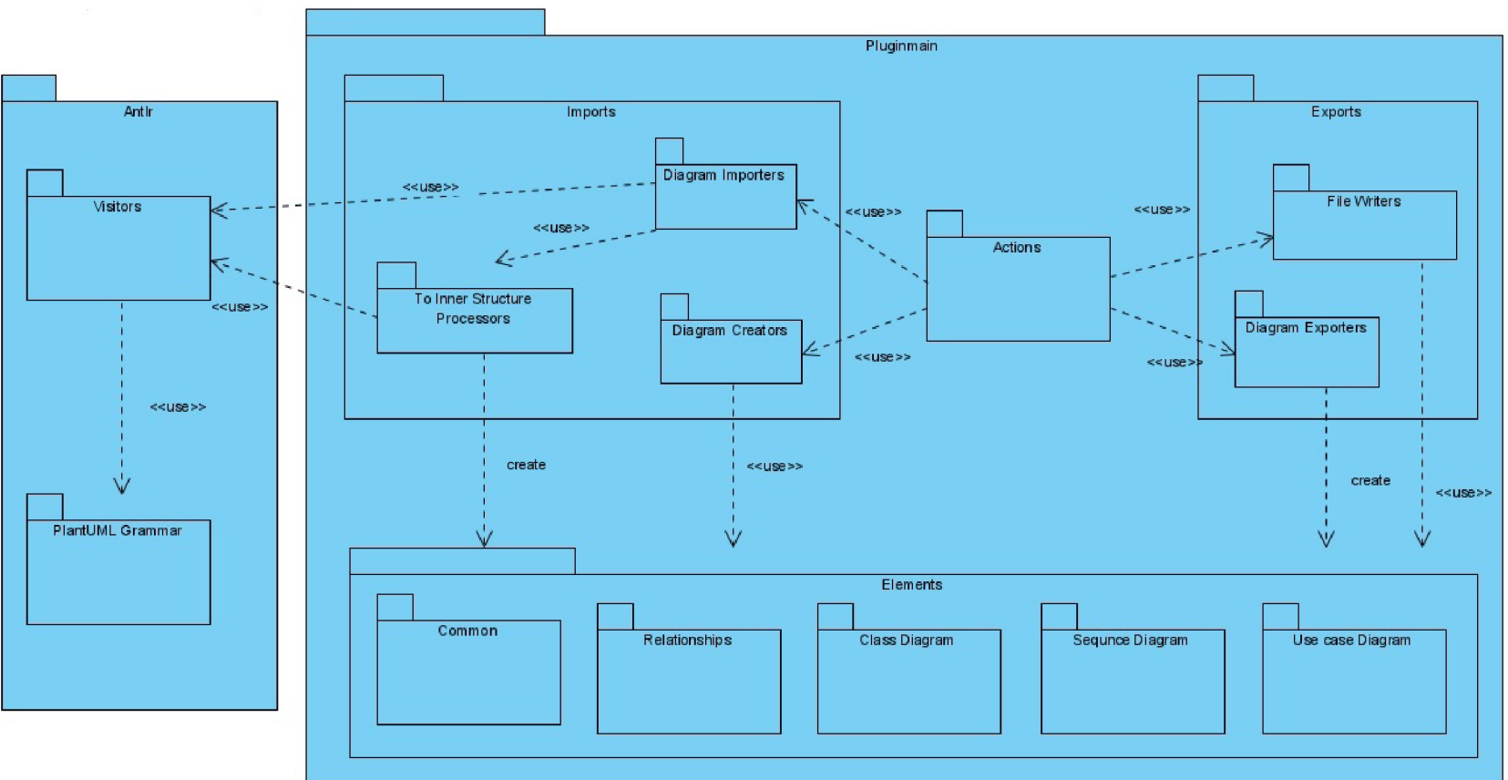
Obrázek 5.4: Zjednodušený package diagram navrženého zástupného modulu
