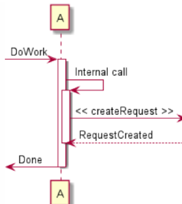
Obrázek 3.10: Příklad sekvenčního diagramu s více čarami života na jednom objektu společně s nalezenými a ztracenými zprávami, převzato z [14]
