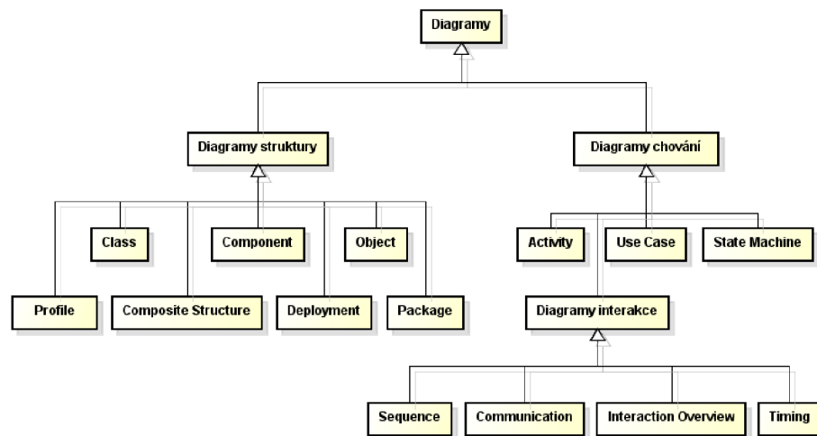
Obrázek 2.1: Struktura zobrazující různé skupiny UML diagramů, převzato z [10]
