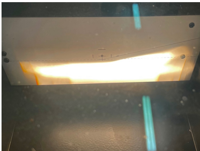
Obrázek 8 - Rozptyl světlometu v regloskopu (Zdroj: Vlastní)
