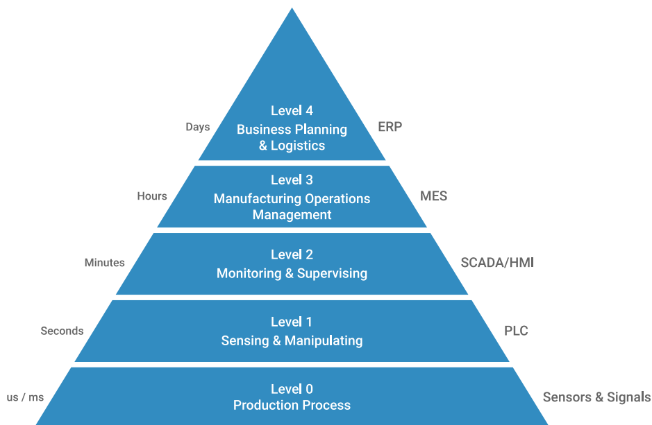
Obrázek 1: Pyramida ISA-95 [2]
