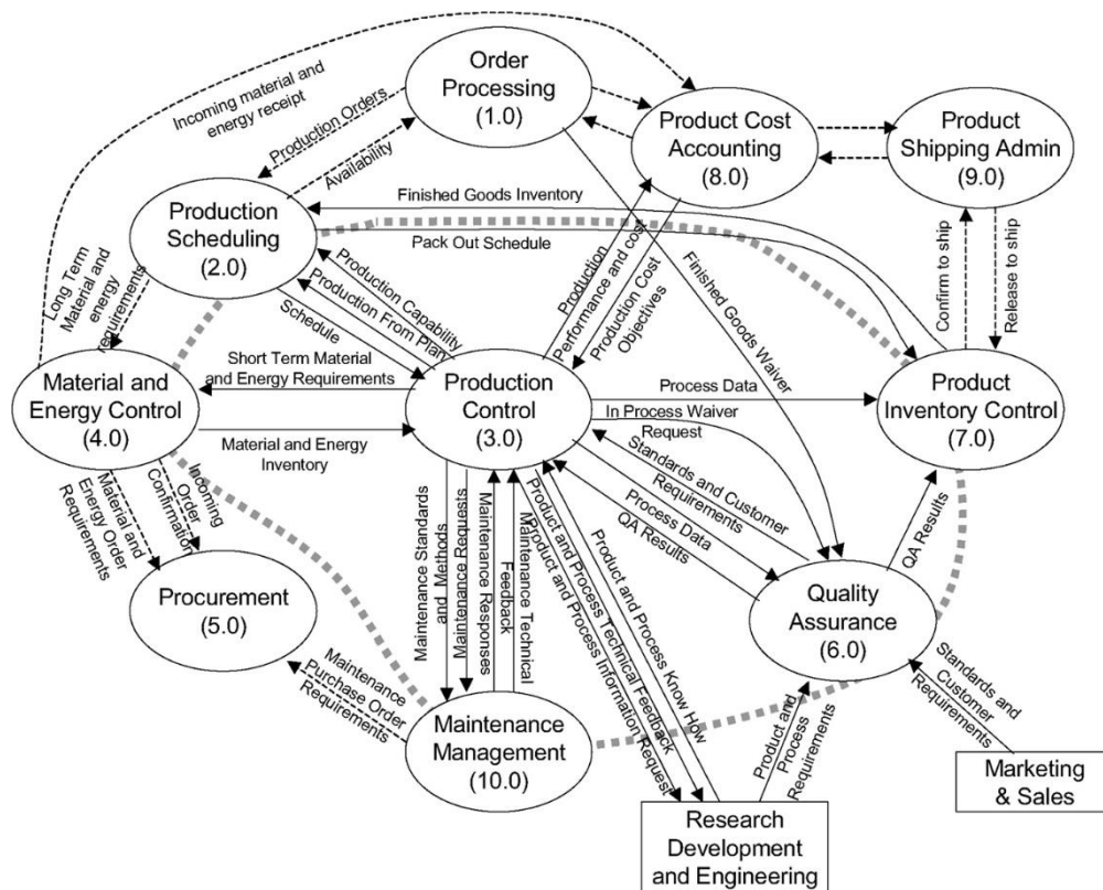
Obrázek 2: Funkcionality ISA-95 [56]
