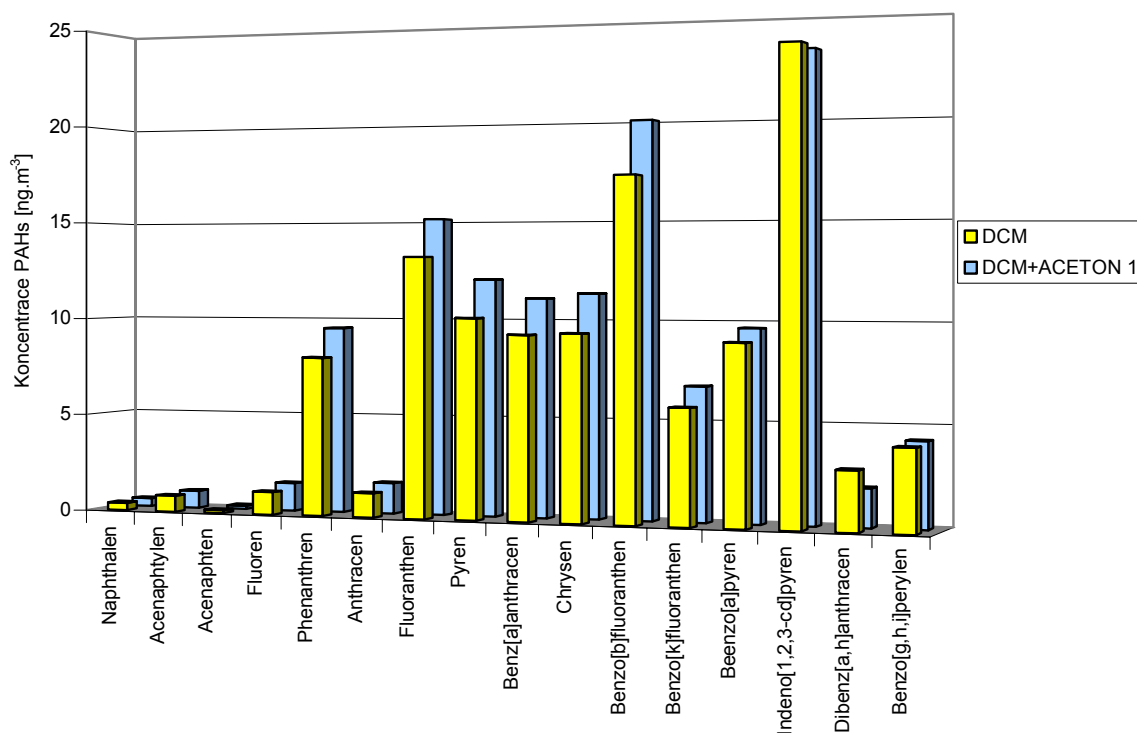
Obr. 5.2.1 – Výtěžnost reálných vzorků u extrakce Soxhlet pro DCM a DCM - aceton
