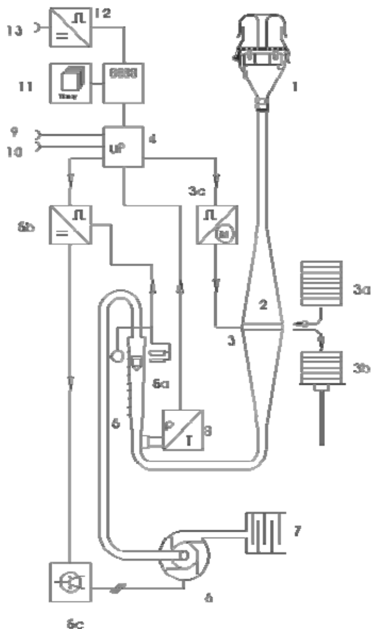
Obr. 4.1.2 – Schéma vzorkovacího zařízení Digital DHA - 80 – (1) PM separátor, (2) průtoková komora, (3) filtr, (3a) zásobník čistých filtrů, (3b) zásobník použitých filtrů, (3c) elektronické zařízení zajišťující automatickou výměnu filtrů, (4) mikroprocesorová kontrola, (5) průtokoměr, (5a) fotosenzor snímající průtok vzduchu, (5b, 5c) kontrolní elektronika, (6) čerpadlo pro nasávání vzduchu, (7) tlumič hluku při výstupu vzduchu, (8) měřicí jednotka tlaku a teploty, (9) výstup pro tisk, (10) rozhraní RS232, (11) slot pro PC kartu, (12,13) vstup pro senzor rychlosti a směru větru(11, 12, 13) jsou nepovinné
