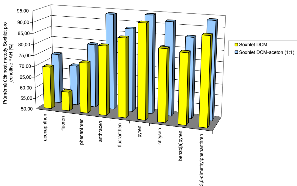
Obr. 5.1.2 – Průměrná účinnost extrakce metody Soxhlet pro jednotlivé PAHs pro DCM a směs DCM – aceton (1:1)
