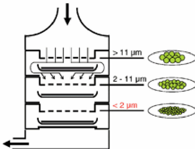
Obr. 2.4.1 – 3-stupňový Andersonův impaktor
