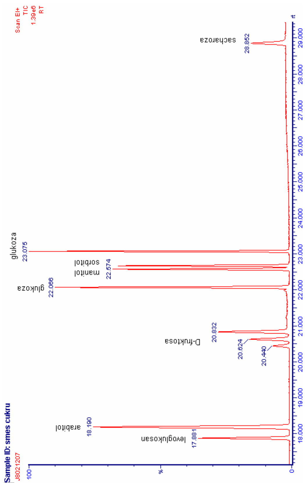
Obr. 9.1.2 – Chromatogram směsi 7 cukrů
