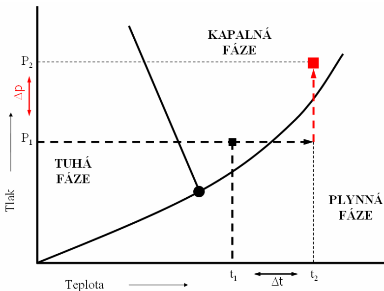
Obr.2.4.3 – Změna stavu rozpouštědla při zvýšení teploty za normálního tlaku a stav rozpouštědla za zvýšené teploty a tlaku
