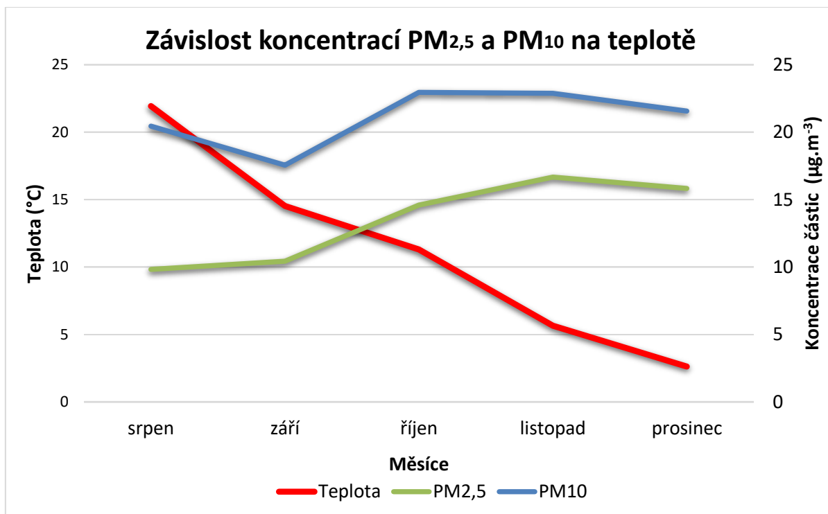
Graf 5 - Závislost koncentrací částic na teplotě. Brno-Úvoz. Roční chod průměrných měsíčních hodnot, srpen až prosinec 2017.
