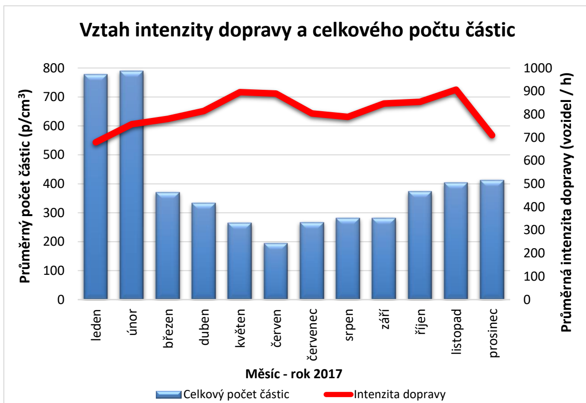
Graf 2 – Závislost intenzity dopravy a celkového počtu částic. Brno-Úvoz. Roční chod průměrných měsíčních hodno), rok 2017.
