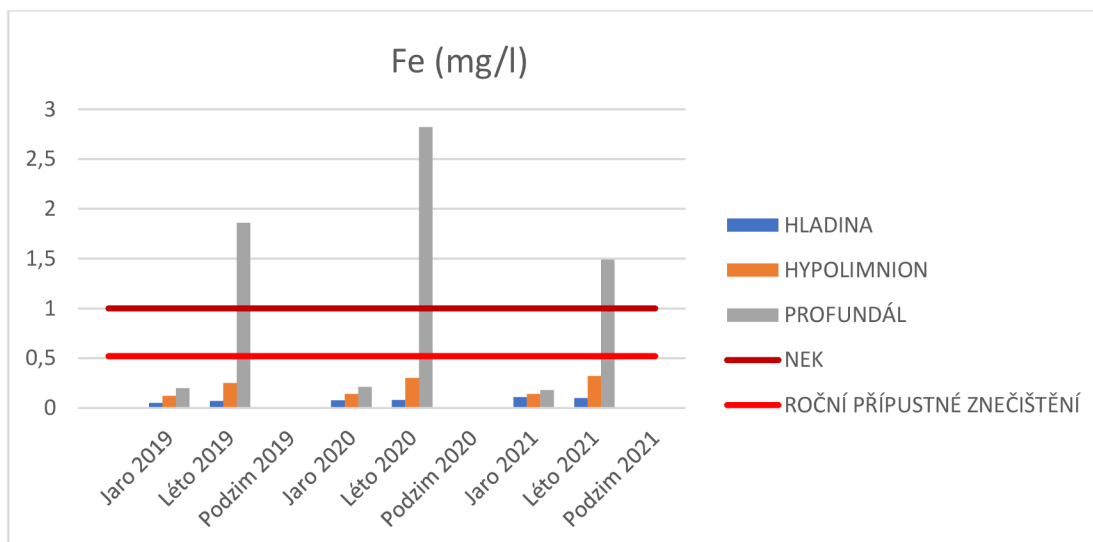
Obrázek 31: Koncentrace železa (Povodí Labe, státní podnik)
