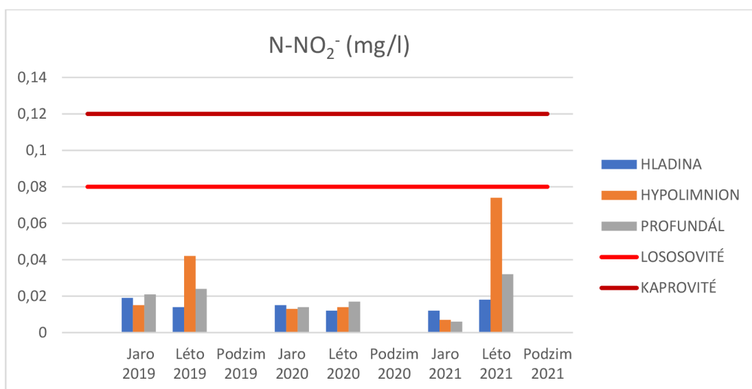
Obrázek 15: Koncentrace dusitanového dusíku (Povodí Labe, státní podnik)
