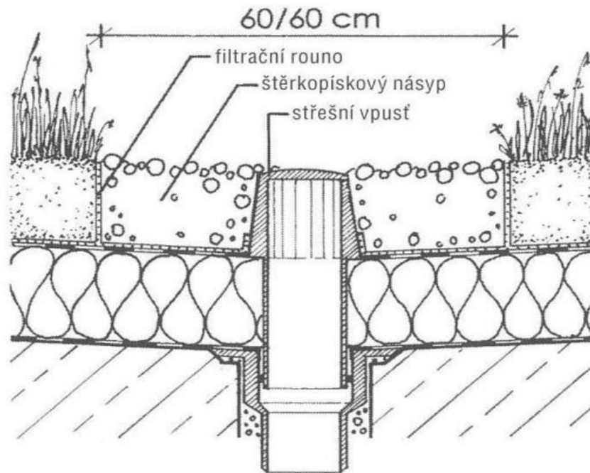
Obrázek 17: řešení vnitřního odvodnění
