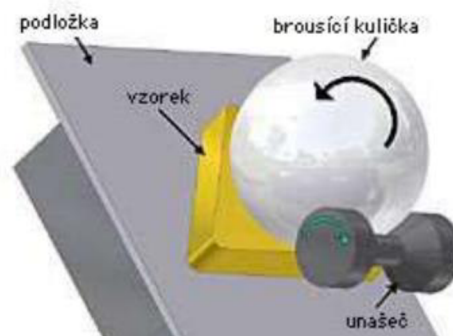
Obr. 14 - Princip kalotestu [3]
