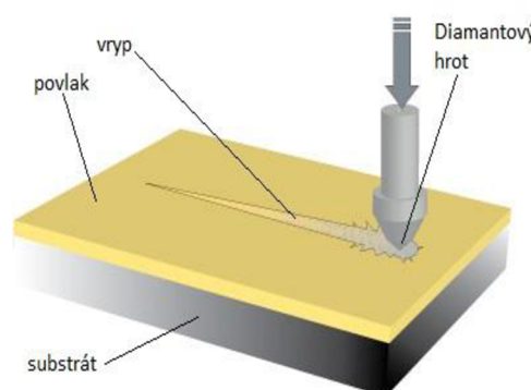
Obr. 15 - Princip scratch testu [7]
