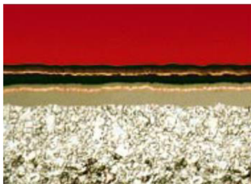
Obr. 24 - Struktura povlaku 6615 [29]
