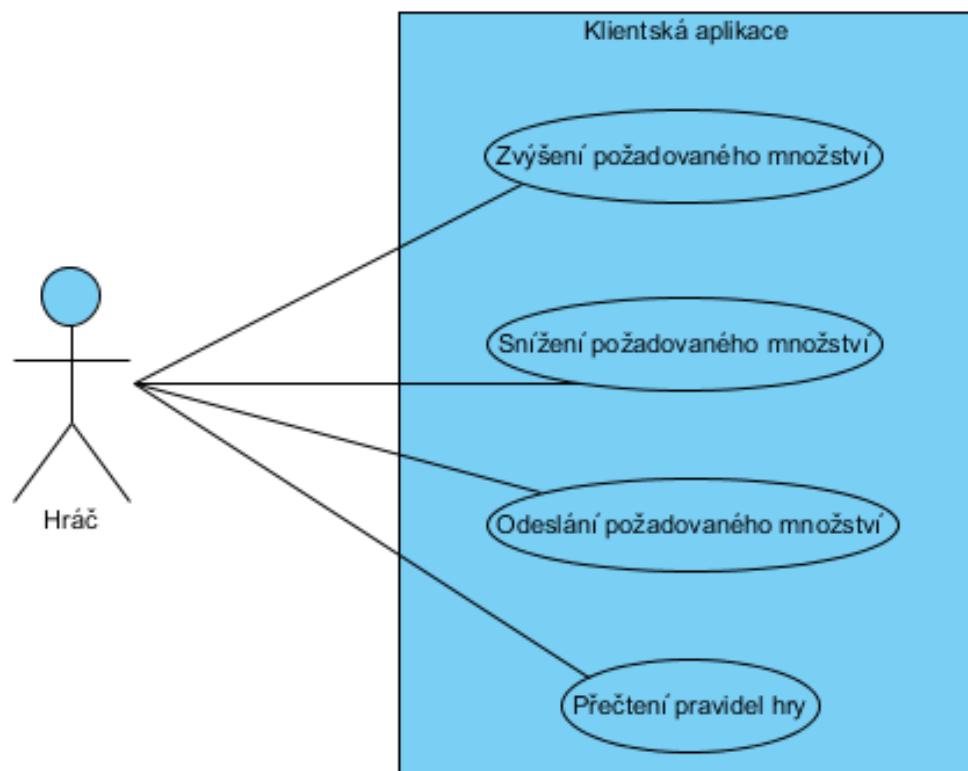
Obr. 8 Usecase diagram hráče a klientské aplikace
