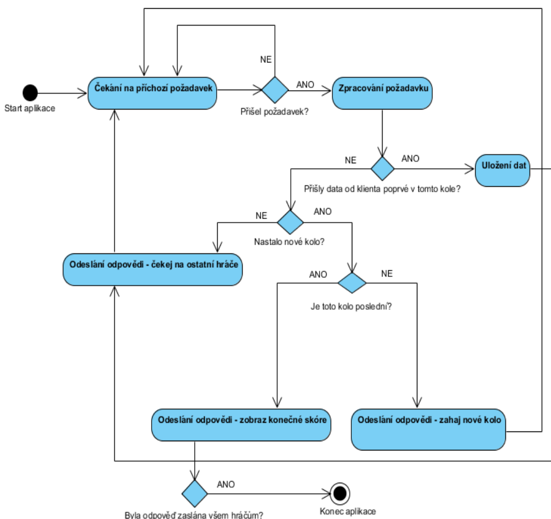
Obr. 6 Diagram aktivit komunikace z pohledu serveru
