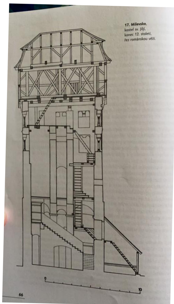
Obr. 25 Řez románskou věží
