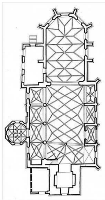
Obr. 242 - Ottensheim, kostel sv. Jiljí, pŕodorys, kolem 1460 - 1510, repro: Bernhard Prokisch, Die Pfarrkirche St. Ägidius in Ottensheim, Oberösterreichische Heimatblätter 1983, č. 2
