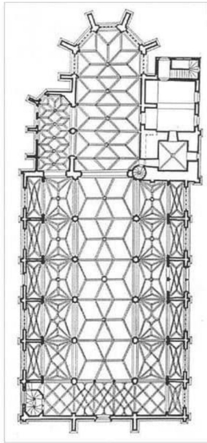
Obr. 243 - Eferding, kostel sv. Hippolyta, púdorys, 1451 - 1497, repro: Bernhard Prokisch, Die Pfarrkirche St. Ägidius in Ottensheim, Oberösterreichische Heimatblätter 1983, č. 2
