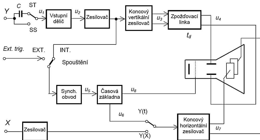
Obr. 1 Blokové schéma analogového osciloskopu. [1]
