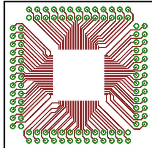
Obr. 12 Návrh redukce TQFP 100 (36x36mm, měřítko 2:1)
