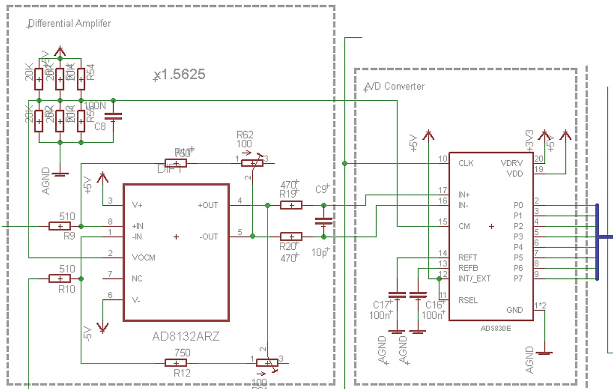
Obr. 18 Diferenční zesilovač a A/D převodník
