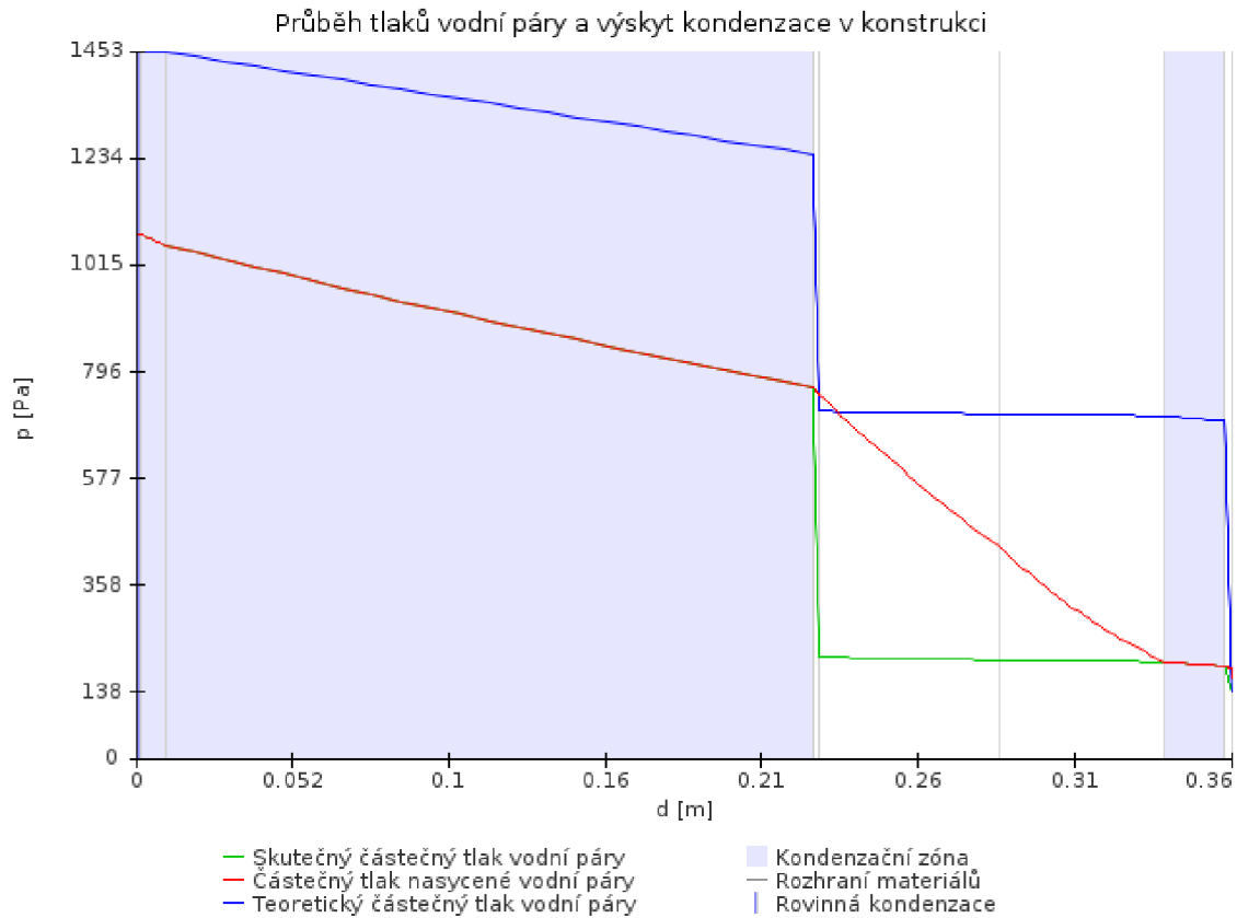
Graf 6 Průběh tlaků vodní páry a výskyt kondenzace v konstrukci
