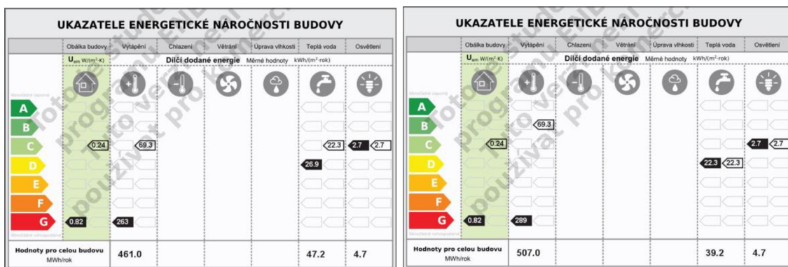
Obrazek 19 Porovnání ukazatelů ENB; teplota vnitřního prostředí 20 °C (vlevo), teplota vnitřního prostředí 21 °C (vpravo)
