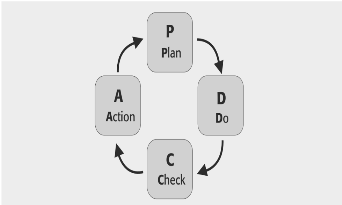
Obrázek 3 Cyklus PDCA
