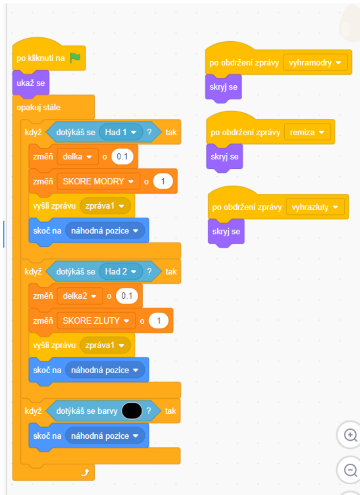
Obrázek 63: Kód postavy Jídlo
