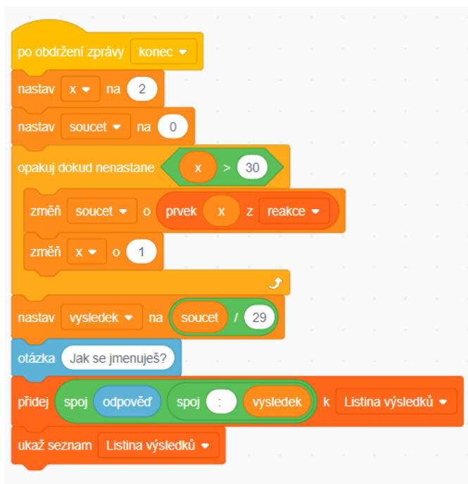
Obrázek 48: Kód postavy Bajtik 2
