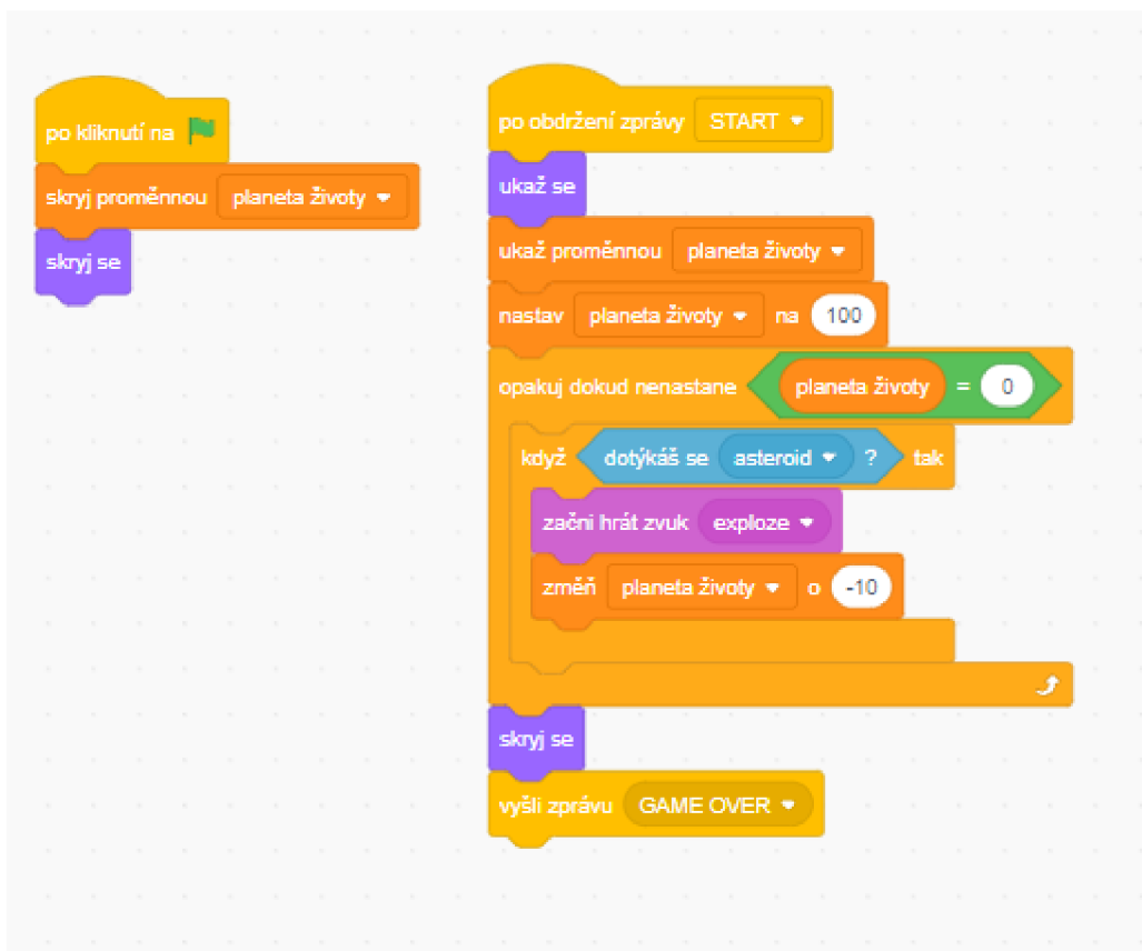
Obrázek 59: Kód postavy planeta
