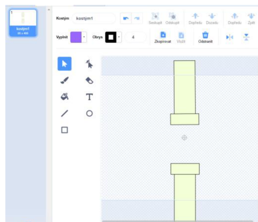
Obrázek 55: Kostým Sloupy
