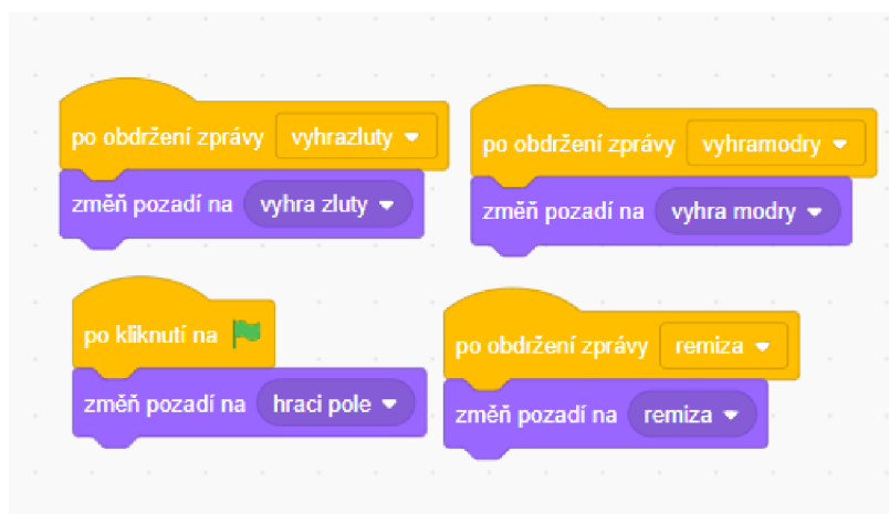
Obrázek 64: Kód pozadí
