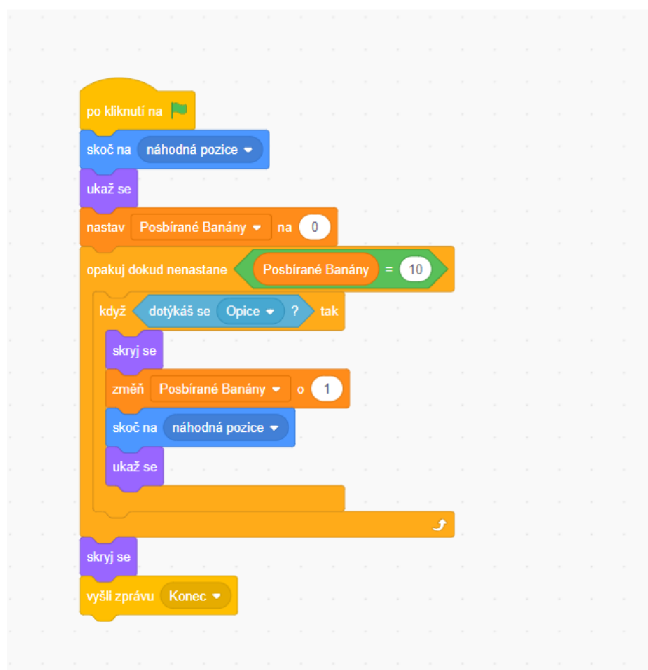
Obrázek 38: Kód Banány
