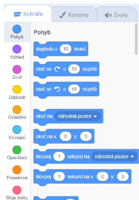
Obrázek 9: Paleta bloků
