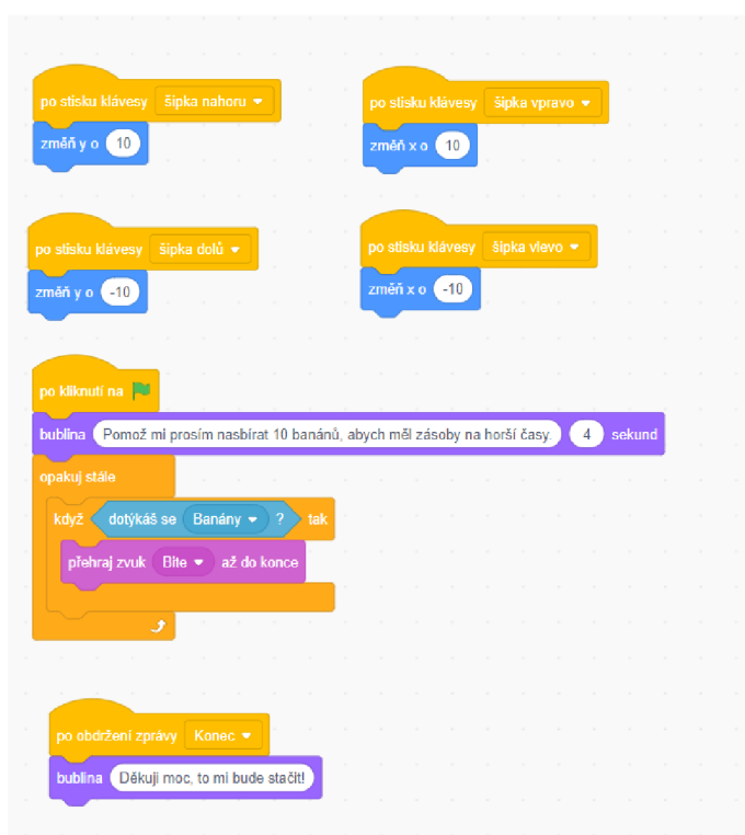
Obrázek 39: Kód Opice
