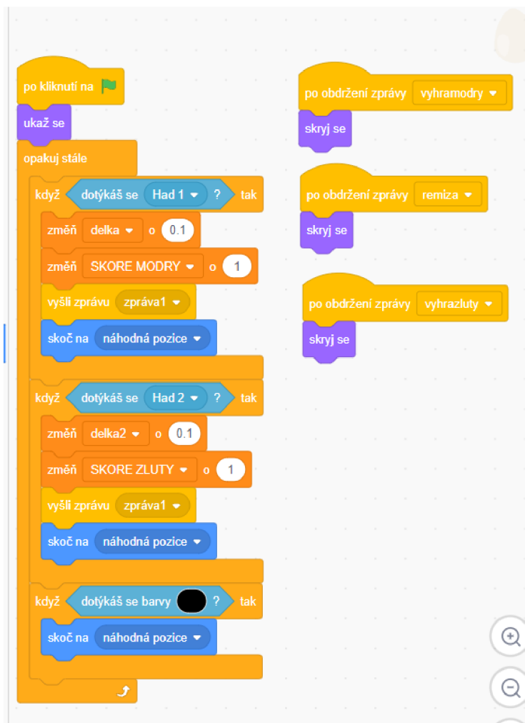
Obrázek 63: Kód postavy Jidlo
