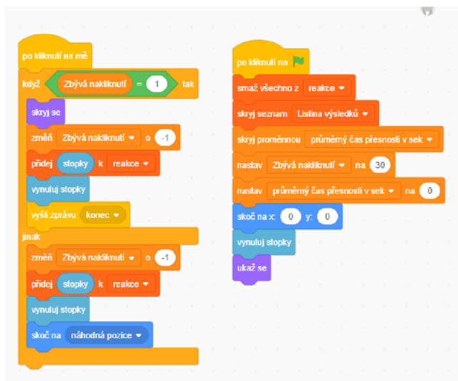
Obrázek 47: Kód postavy Bajtik 1
