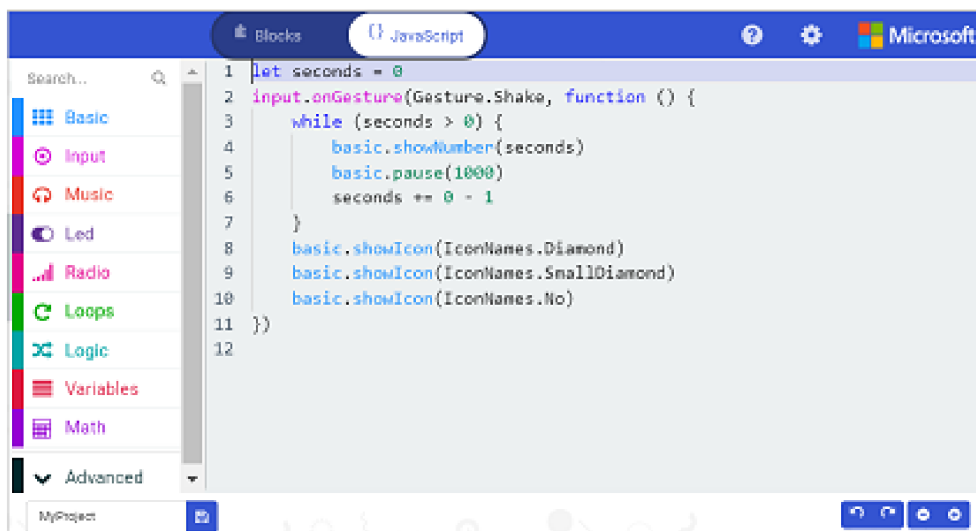
Obrázek 15: Jazykový editor v MakeCode, převod bloků do JavaScriptu 9
