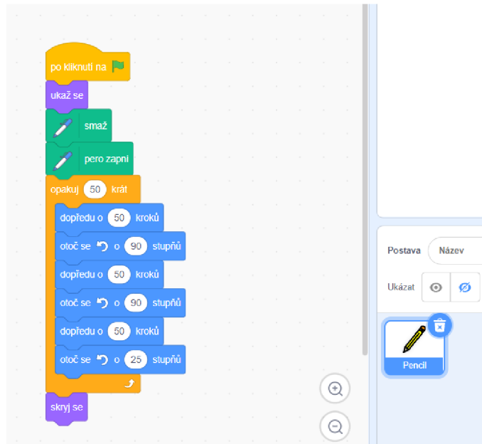
Obrázek 28: Kód pro vytvoření Mandaly
