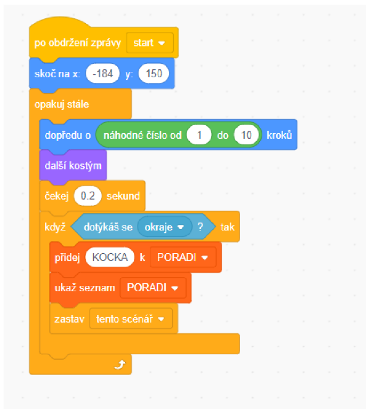
Obrázek 40: Kód Kočka
