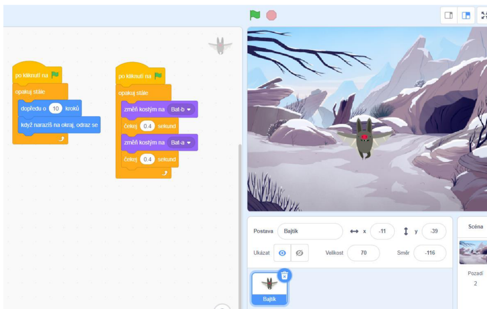
Obrázek 17 Kód Bajtik
