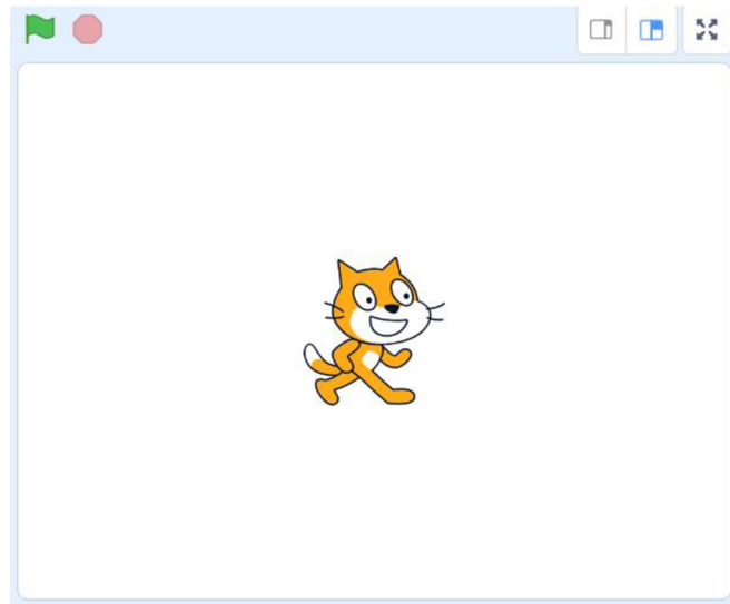
Obrázek 7: Scéna programu
