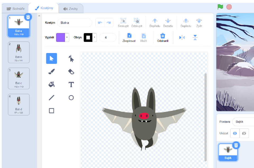
Obrázek 18 Postava Bajtik
