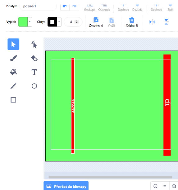
Obrázek 42: Pozadí
