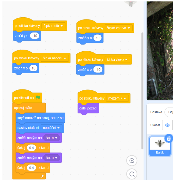
Obrázek 20: Kód Bajtik
