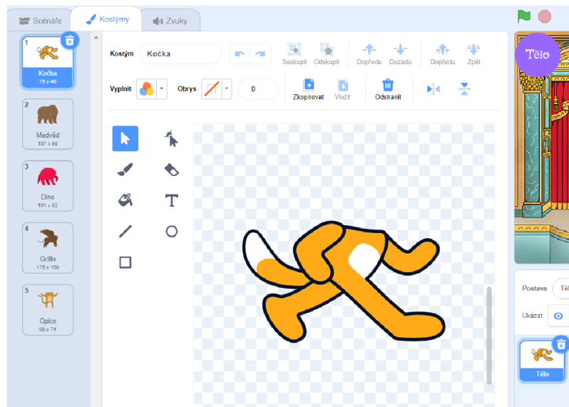
Obrázek 27: Kostýmy Tělo
