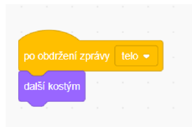
Obrázek 24: Kód Tělo
