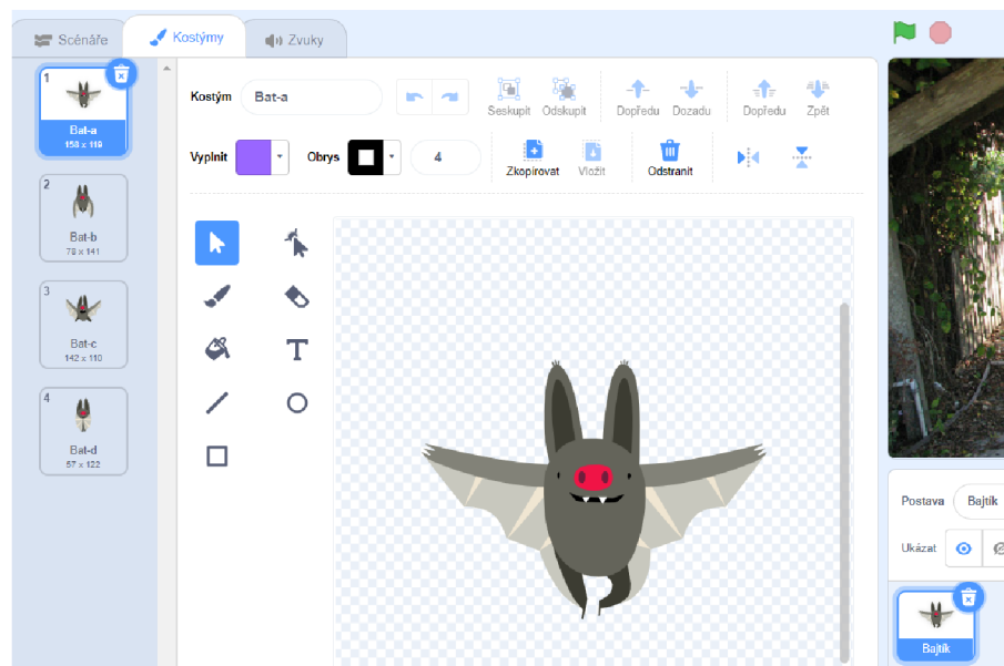
Obrázek 21: Kostým Bajtik
