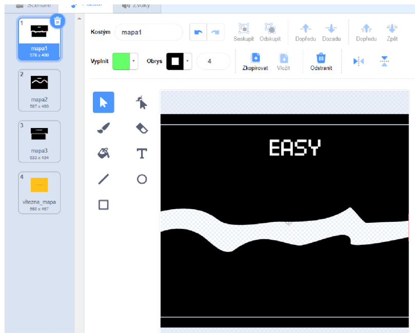
Obrázek 44: Ukázka dráhy
