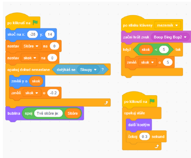
Obrázek 53: Kód postavy Bajtik
