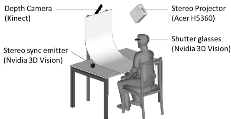
Obrázek 2.4: Systém MirageTable [7].
