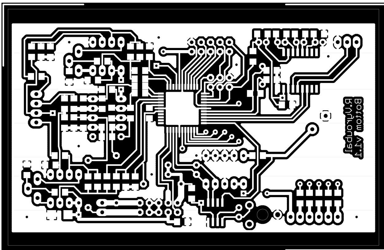
Obr. 40.: DPS řídicí jednotky BOTTOM (spodní strana, rozměry 100 x 63,5)
