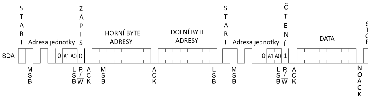
Obr. 18.: Čtení jednoho byte
