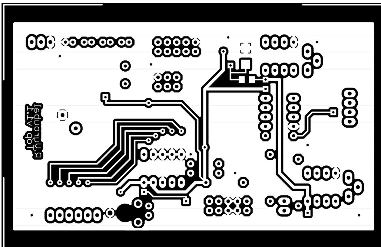
Obr. 41.: DPS řídicí jednotky TOP (spodní strana, rozměry 100 x 63,5)
