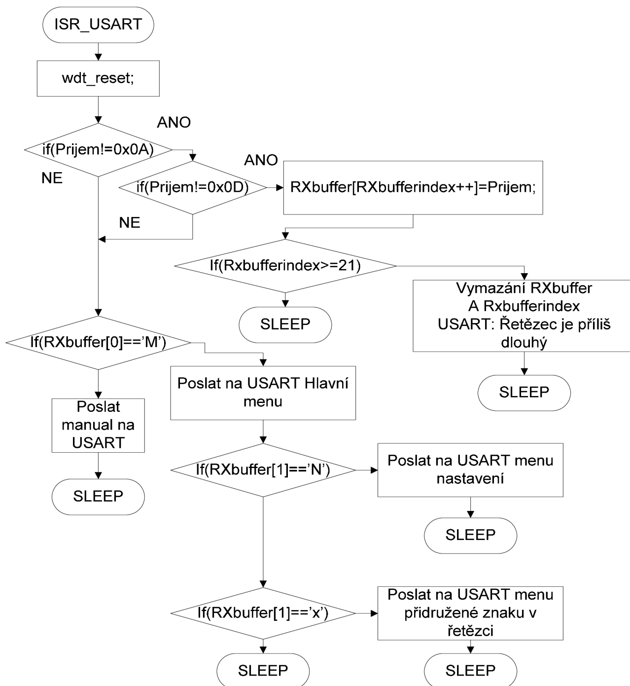
Obr. 50.: Vývojový diagram přerušeni od jednotky USART
