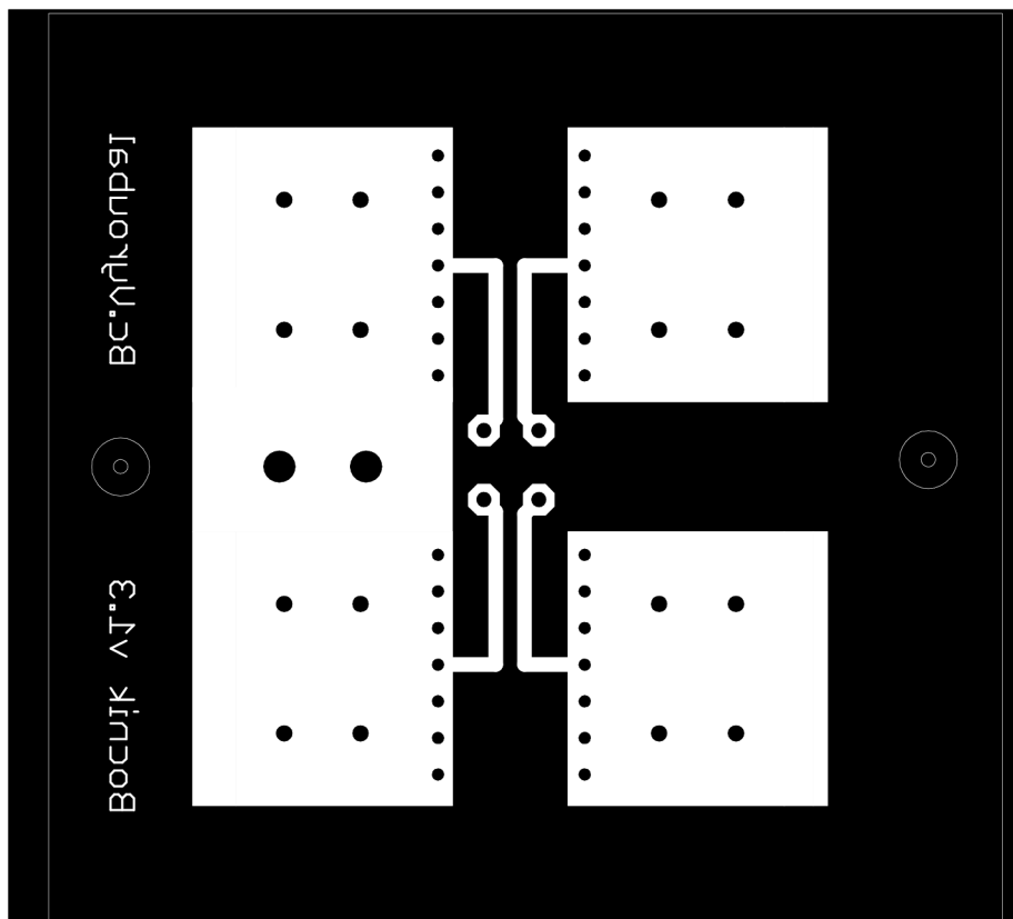
Obr. 37.: DPS bočníků (rozměry 66 x 63)
