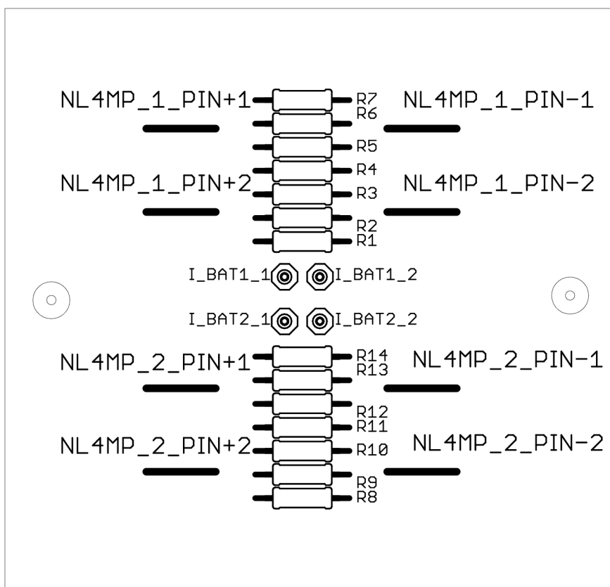
Obr. 38.: Osazovací plán bočníků TOP, odpory substituují odporový drát.
