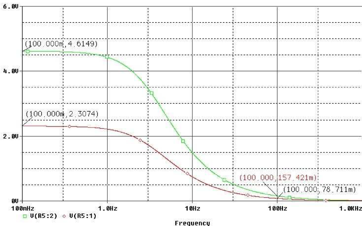
Obr. 11.: Frekvenční charakteristika diferenčního operačního zesilovače pro měření proudu (zelený marker odpovídá MALE_I na Obr. 10, červený VELKE_I)
