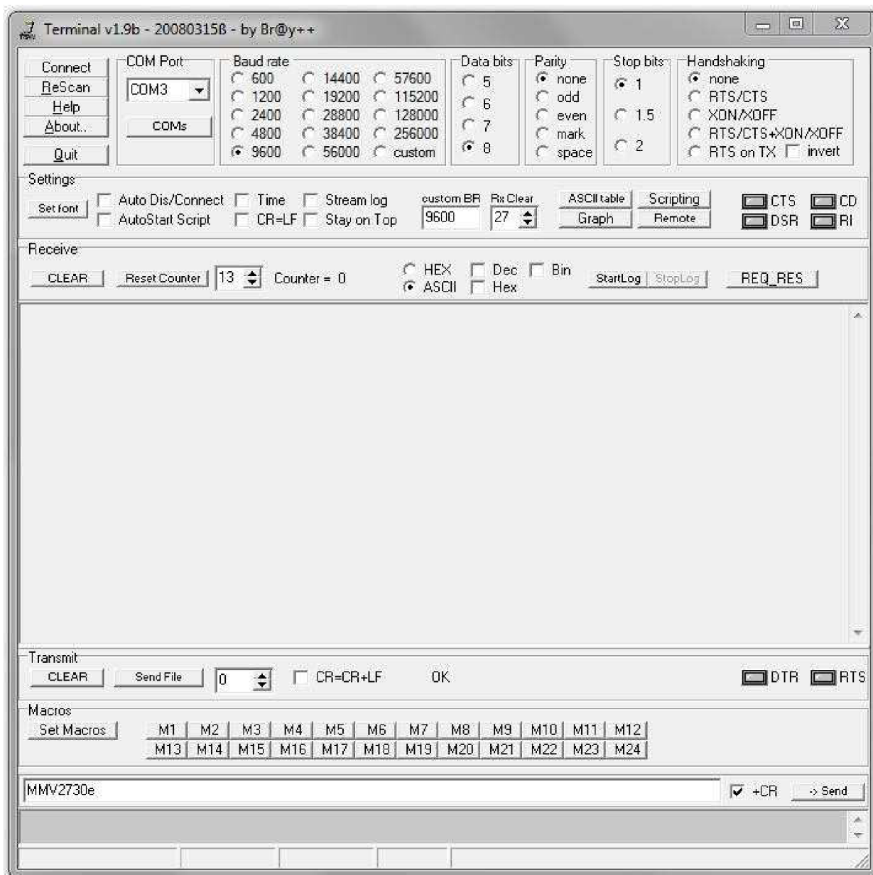
Obr. 58.: Nakonfigurovaný terminál
