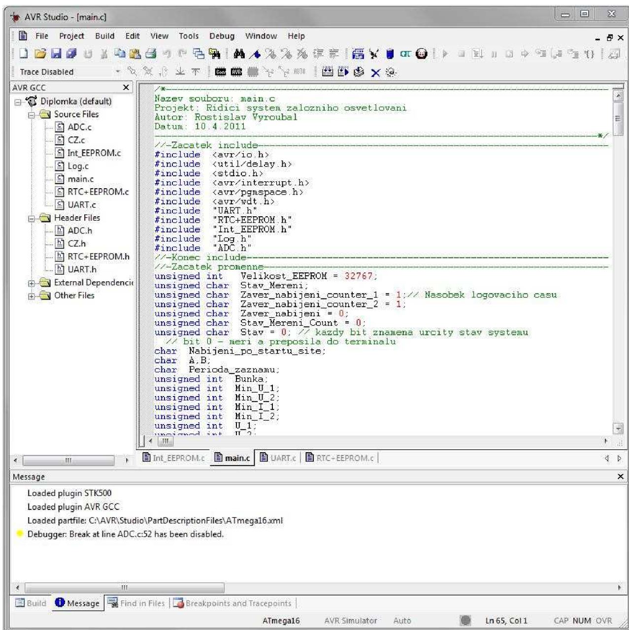
Obr. 54.: AVR Studio
