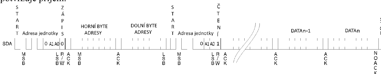
Obr. 19.: Sekvenční čtení
