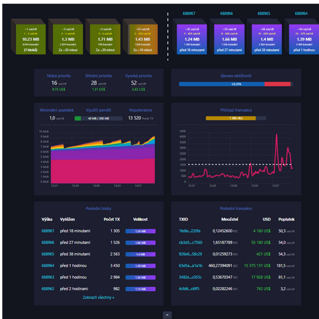
Obrázek 1: Mempool
