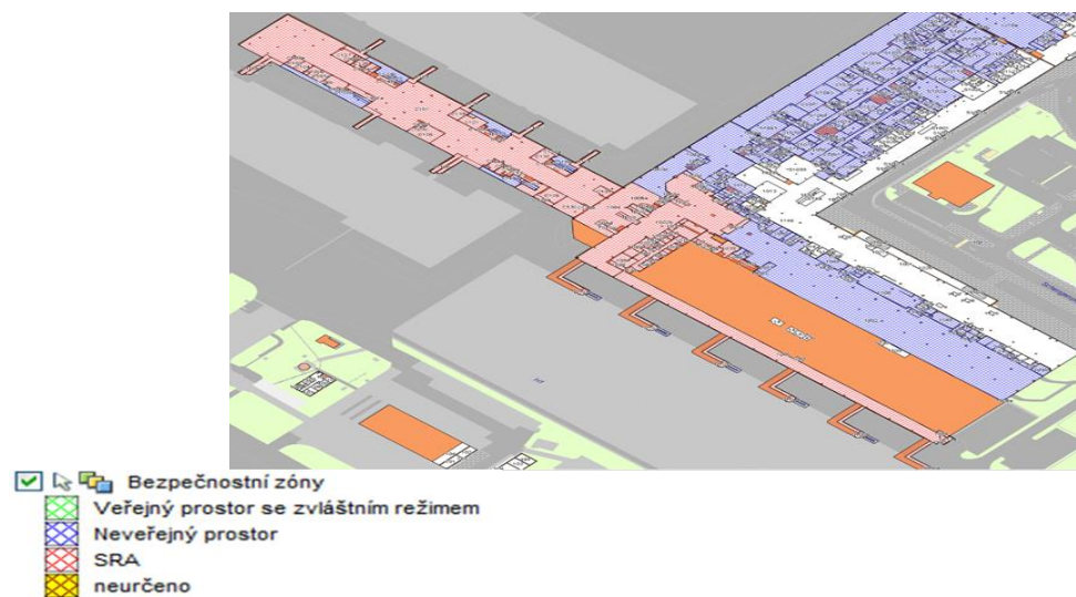
Obrázek 11: Bezpečnostní zóny Terminál 2
