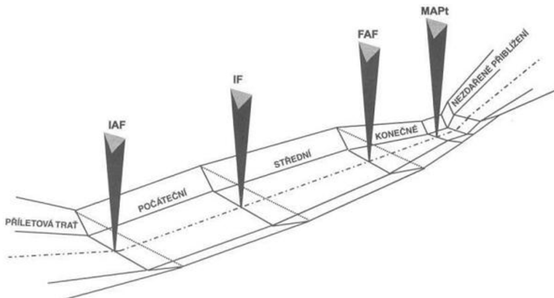
Obr. 3: Úsek příletové trati a úseky přiblížení oddělené fixy [2]
