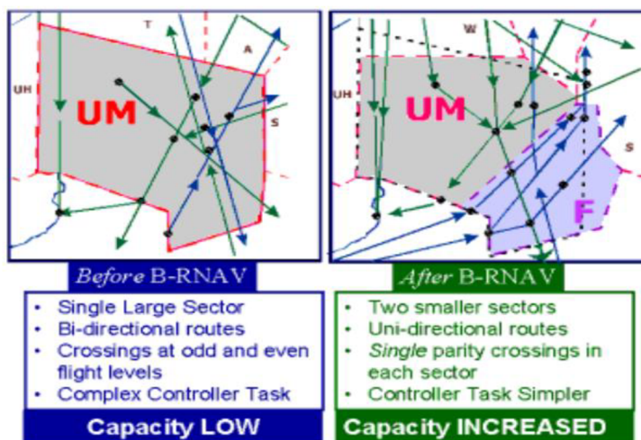
Obr. 4: Srovnání využitelnosti provozu v segmentu bez B-RNAV a s použitím B-RNAV [7]
