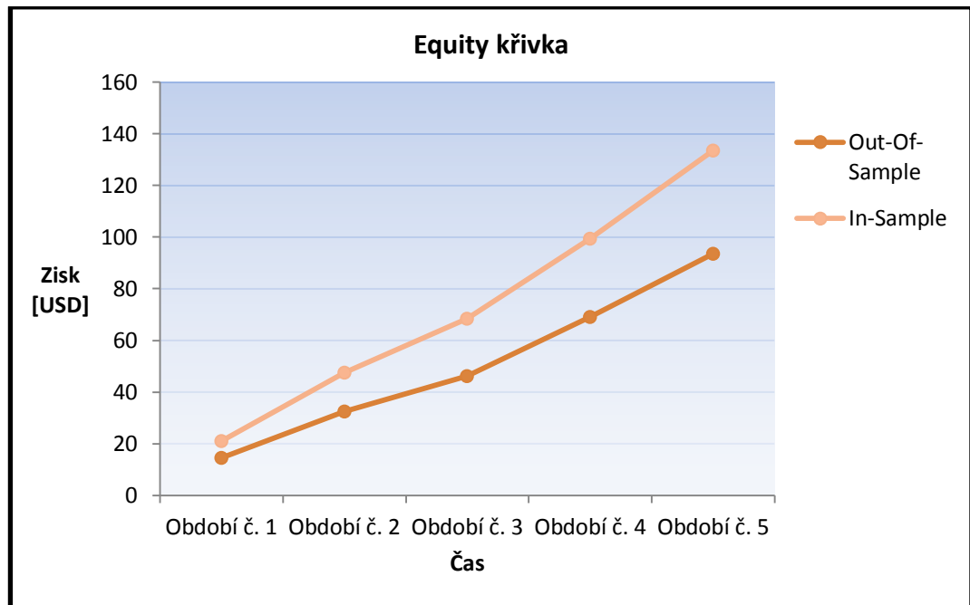
Graf č. 10: Equity křivka napříč obchodních období
