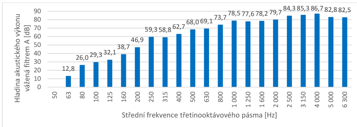
Obr. 27 Hladiny akustického výkonu vážené funkci A pro jednotlivá frekvenční pásma
