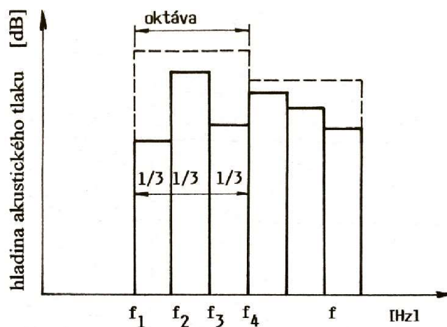
Obr. 4 Třetinooktávové pásmo [3]
