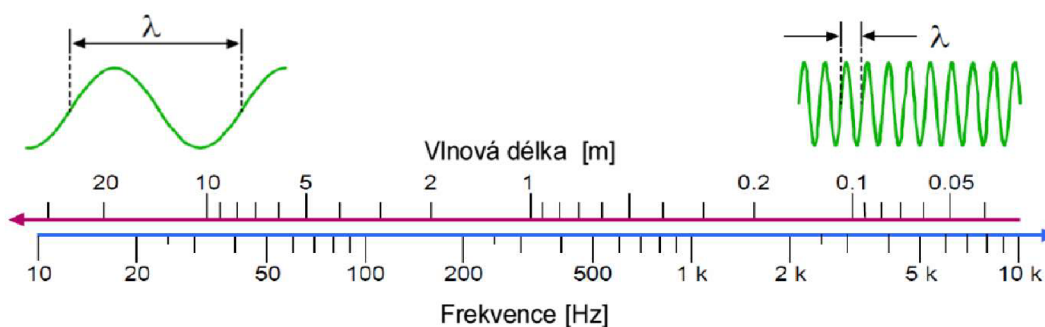
Obr. 6 Vlnová délka [7]
