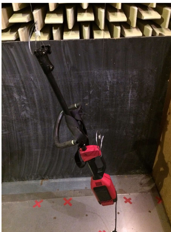
Obr. 17 Způsob zavěšení zdroje hluku
