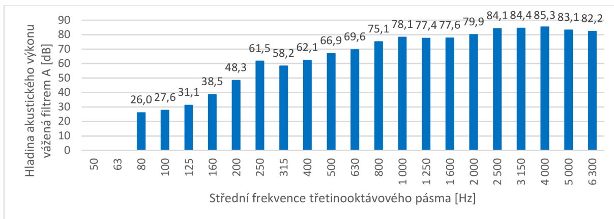
Obr. 25 Hladiny akustického výkonu vážené funkci A pro jednotlivá frekvenční pásma
