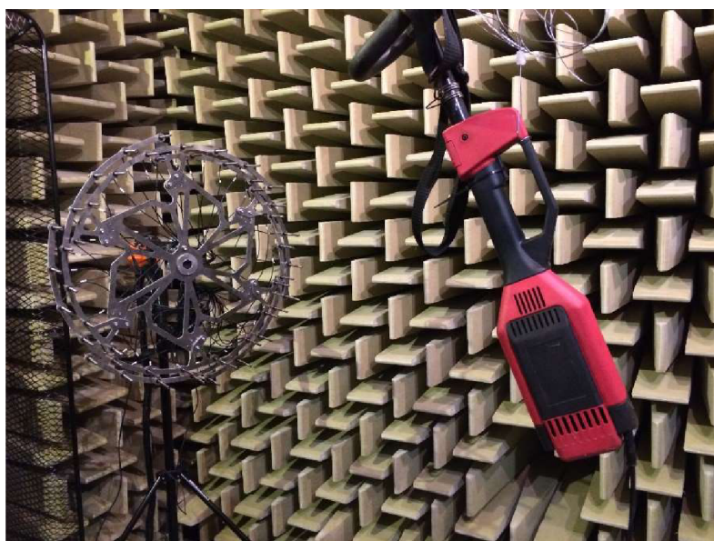
Obr. 32 Lokalizace zdroje hluku pomocí akustické kamery
