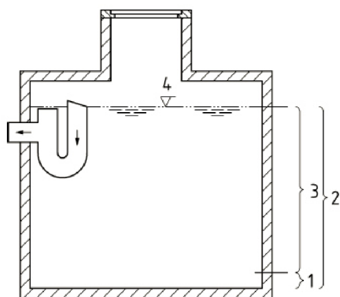
Obr. 16: Objem akumulční nádrže [2]
