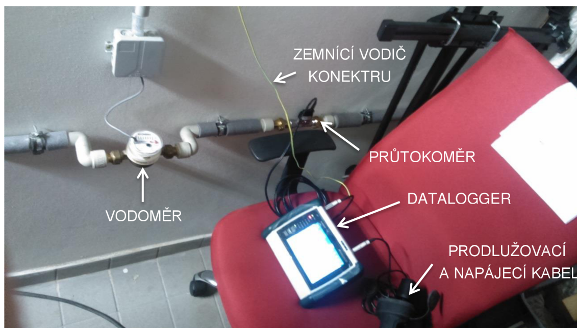
Obr. 27: Umístění měřicího zařízení (AB)
