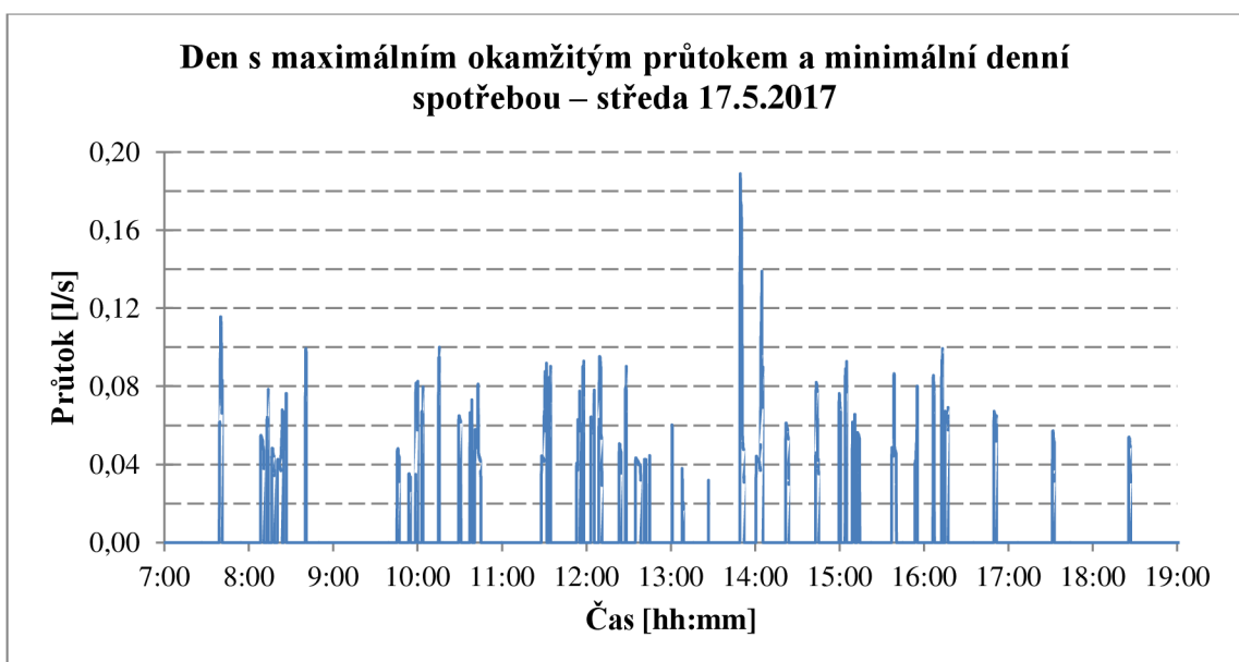
Graf 9: Kontinuální zobrazení průtoku 2 (AB)
