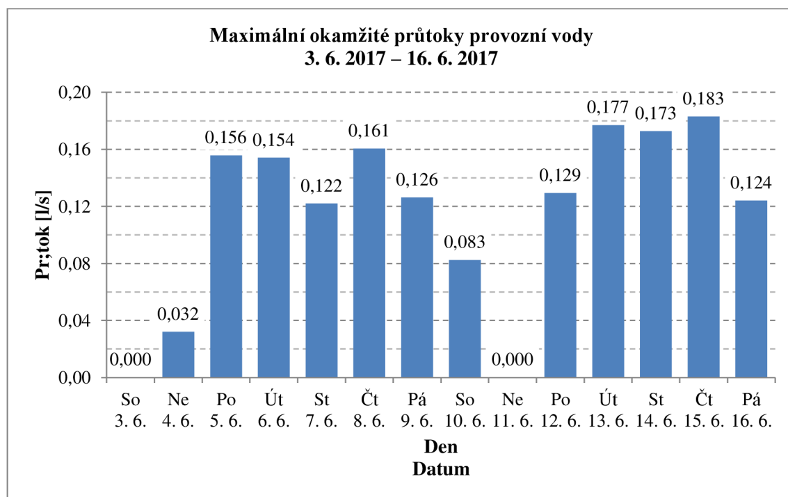
Graf 15: Maximální okamžité průtoky provozní vody (VaVC)
