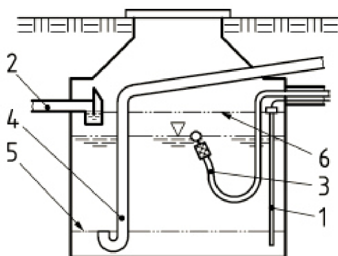
Obr. 13: Příklad vybavení akumulární nádrže pro čerpadlo umístěné mimo nádrž [2]
