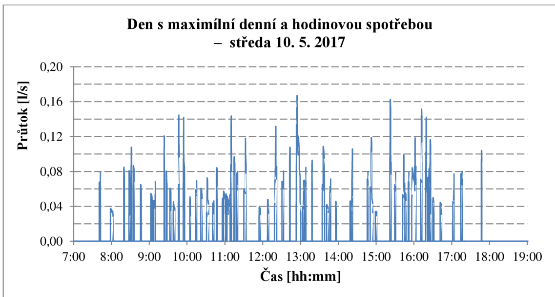
Graf 8:Kontinuální zobrazení průtoku 1 (AB)
