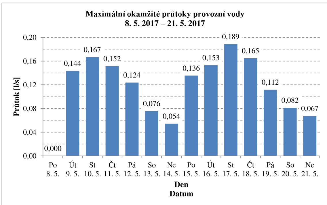
Graf 7: Maximální okamžité průtoky provozní vody (AB)
