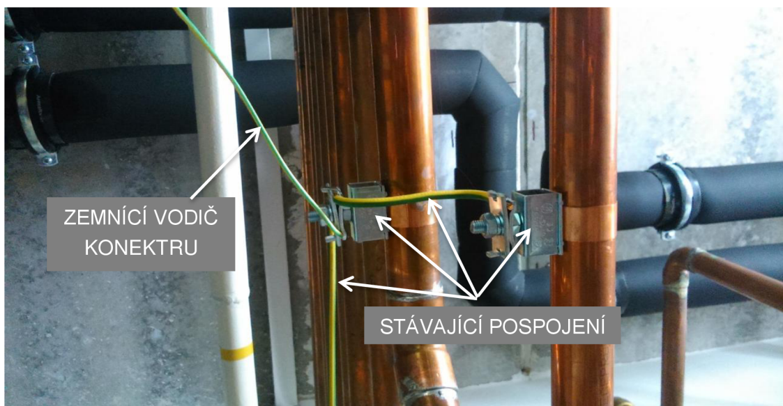
Obr. 29: Pospojení konektoru snímače průtoku (AB)
