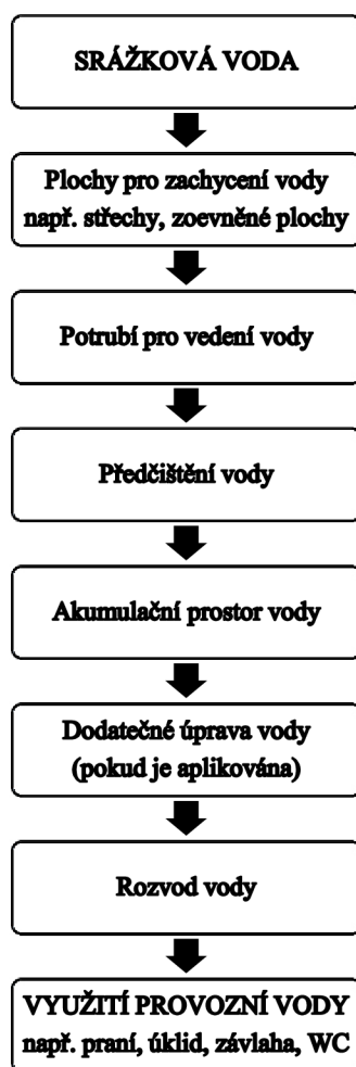
Obr. 1: Cesta od srážkové vody k provozní
