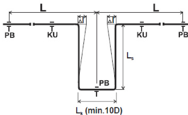
Obr. 39 U kompenzátor [15]
