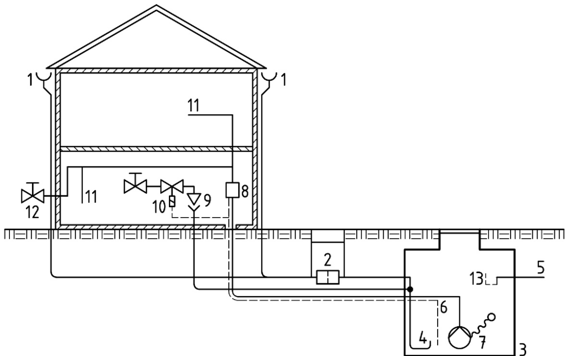
Obr. 9: Systém s doplňováním vody do akumulční nádrže [2]
