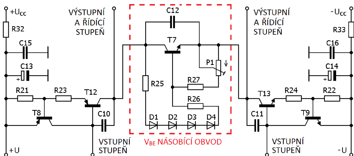
Obr. 7: Schéma zapojení druhého stupně
