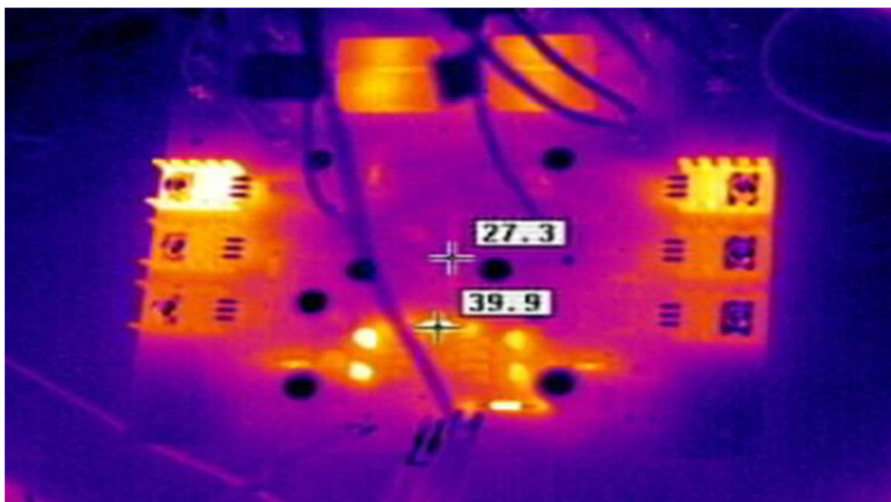
Obr. 26: Deska plošných spojů výkonového zesilovače vyfocena termokamerou
