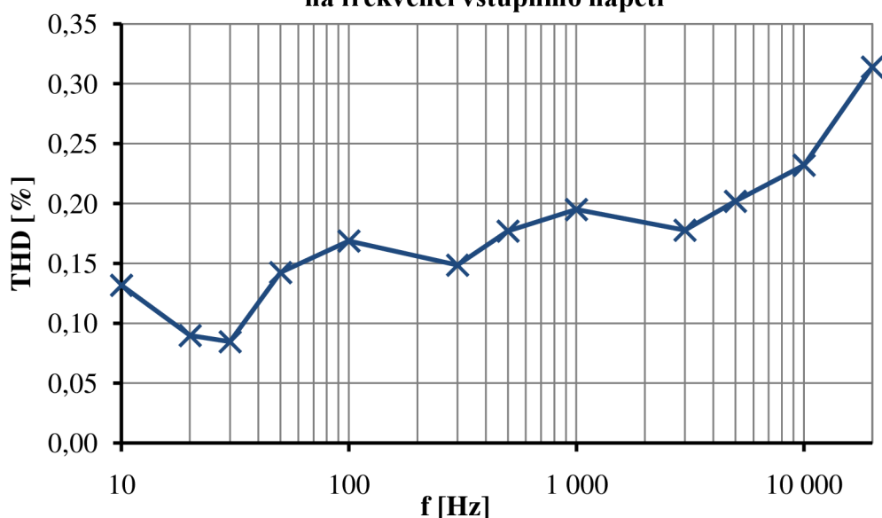
Zkreslení THD výkonového zesilovače v závislosti na frekvenci vstupního napětí
