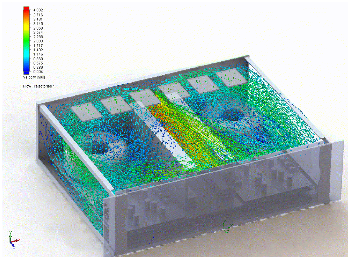
Obr. 35: Proudění uvnitř zesilovače při použití jednoho ventilátoru
