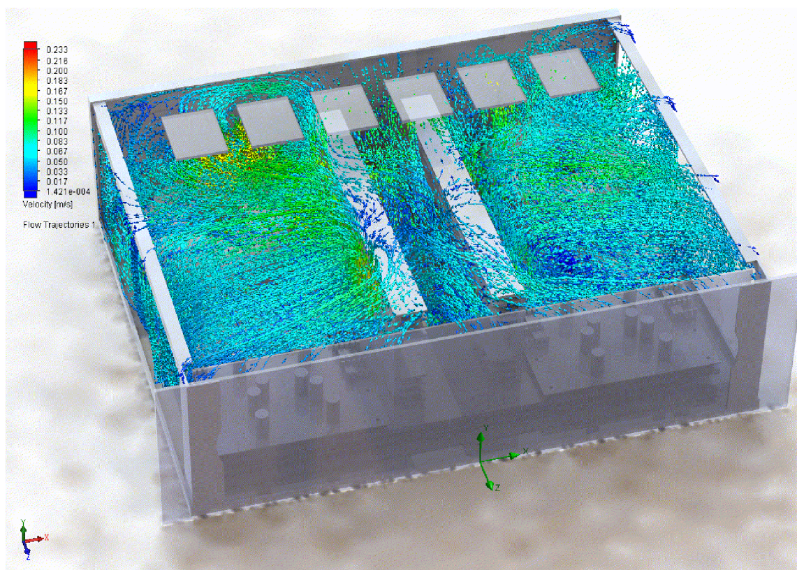
Obr. 33: Proudění vzduchu uvnitř zesilovače bez použití ventilátorů
