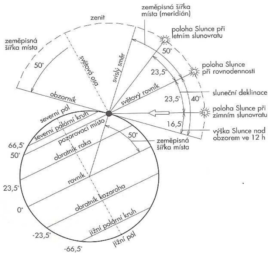
Obr. 2.3: Sluneční souřadnice a pohyb Slunce po obloze.
