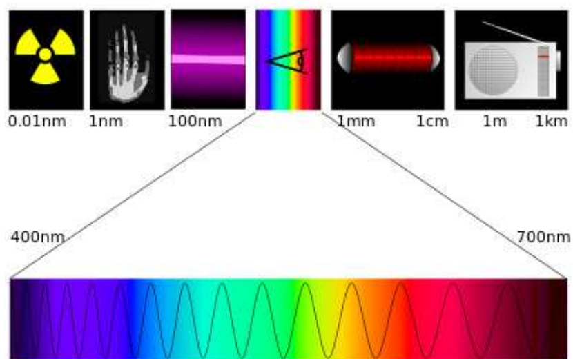
Obr. 2.4: Spektrum vlnových délek
