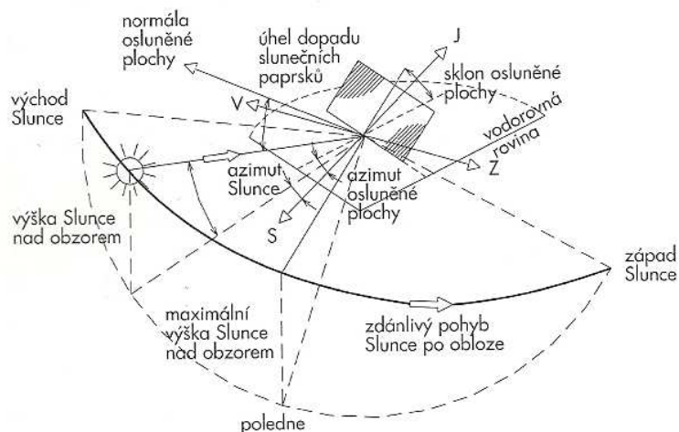
Obr. 2.2: Sluneční souřadnice na obloze a osluněné plochy
