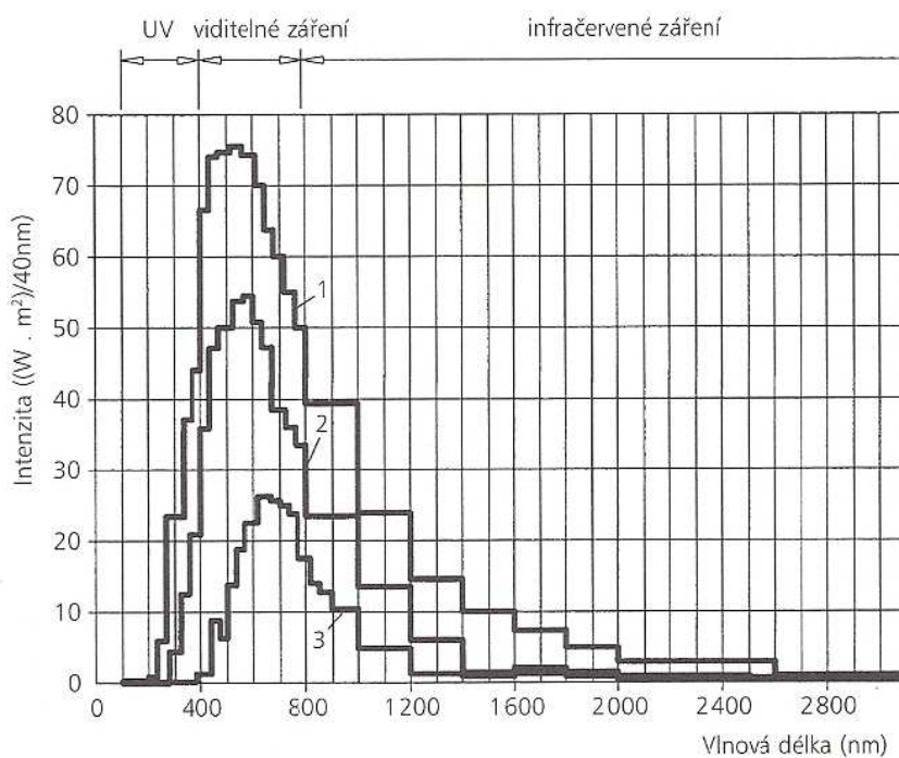
Obr. 2.5: Spektrální rozdělení energetického obsahu slunečního záření
