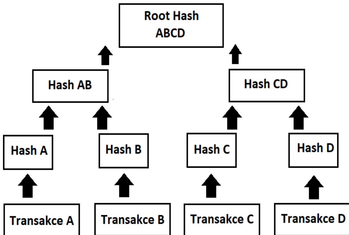
Obr. 2.2 Merklův strom
