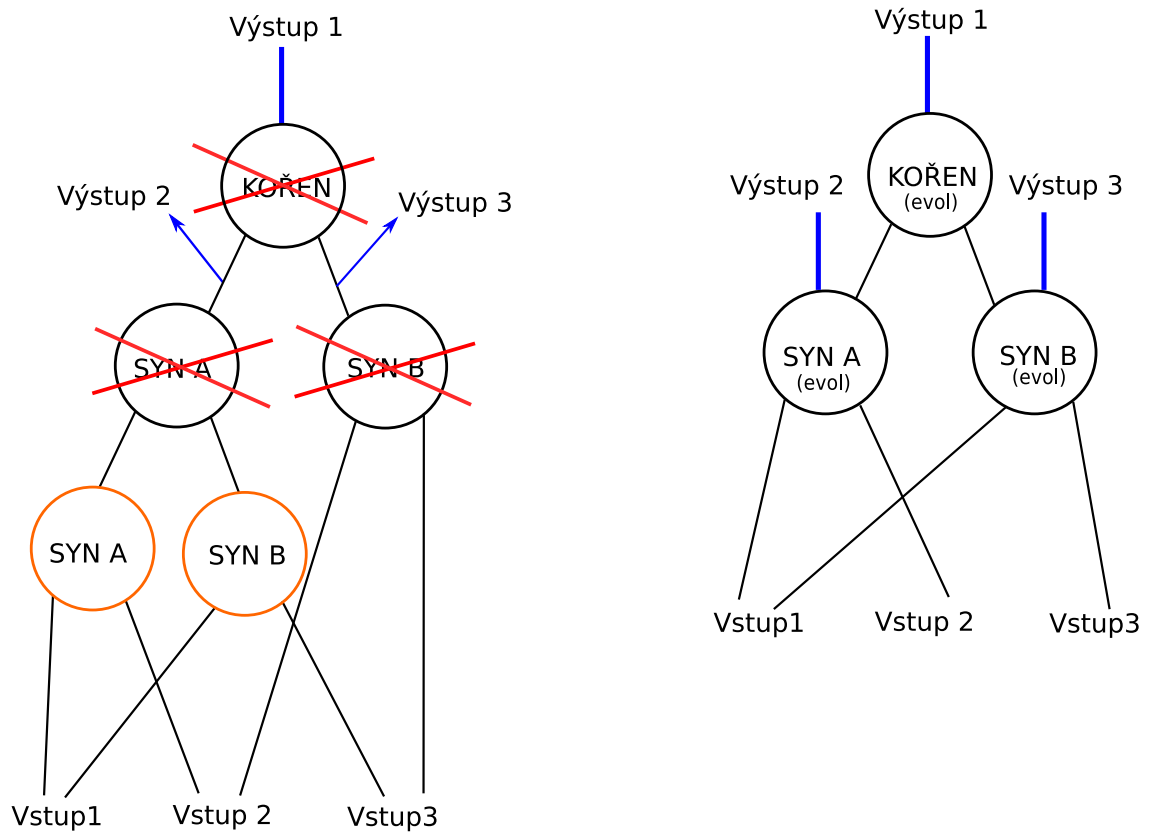
Obrázek 3.9: Vlevo je původní řez s modře vyznačenými výstupy. Vpravo je evolvovaný řez se stejným počtem výstupů napojených na původní výstupní rozhraní. Vstupy, využívané řezem vlevo, jsou také využity. Červeně přeškrtnutá hradla jsou odstraněna a nahrazena odpovídajícími evolvovanými hradly v obvodu vpravo. Oranžová hradla jsou ponechána v původním obvodu a po skončení rozšíření případně vyoptimalizována Yosysem.
