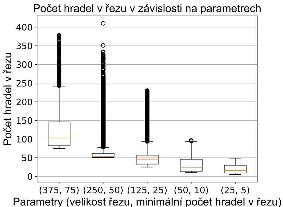
Obrázek 4.1: Znárodnění statistického rozložení hodnoty počtu hradel v řezu v závislosti na daných parametrech.
