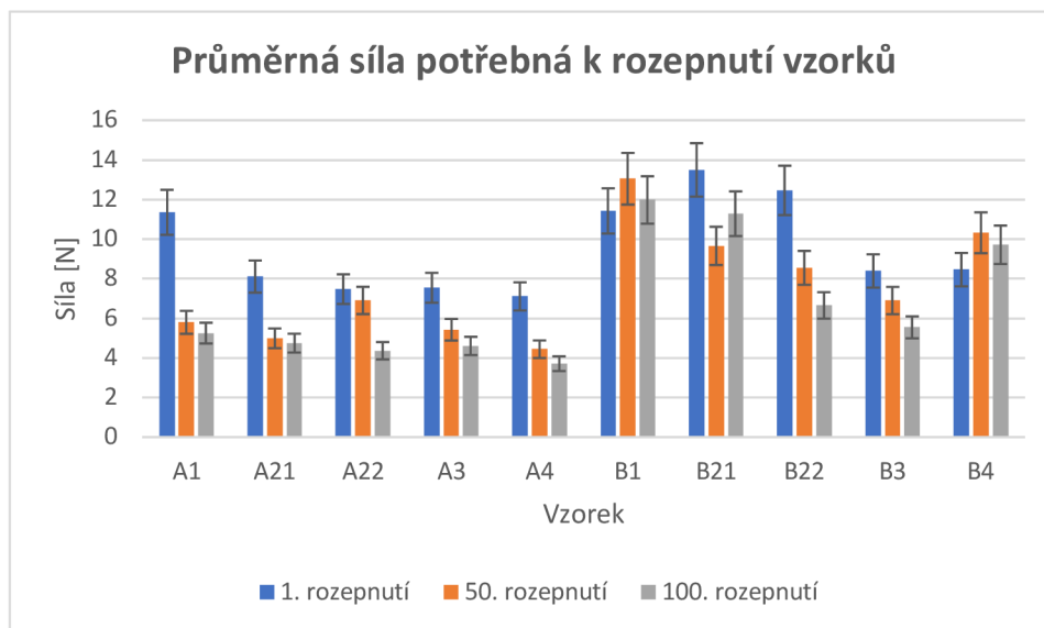
Graf 13 Průměrná síla potřebná k rozeptutí vzorků
