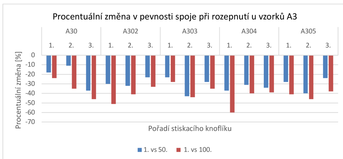
Graf 6 Procentuální změna v pevnosti spoje při rozepnutí u vzorků A3
