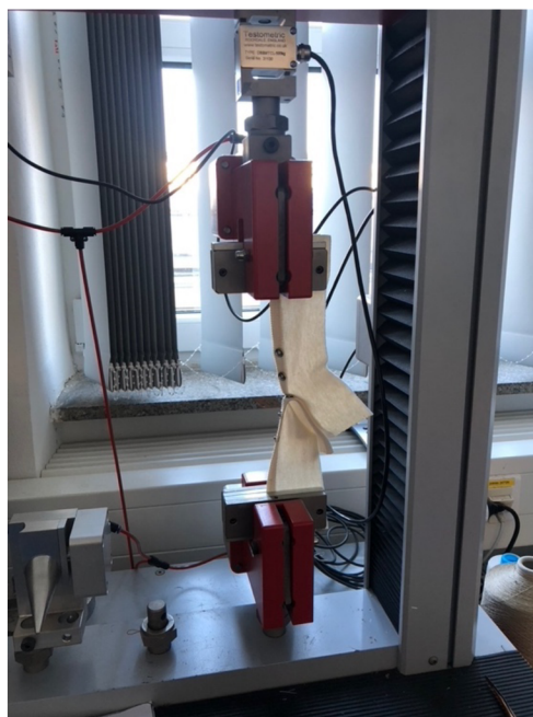
Obrázek 31 Trhací stroj Testometric [vlastní zdroj]
