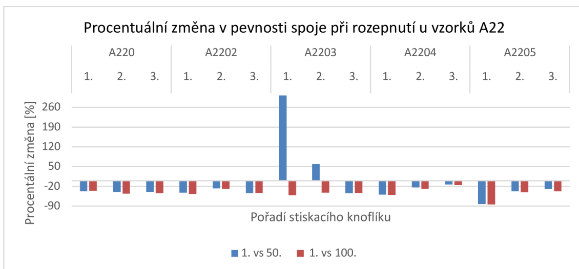
Graf 5 Procentuální změna v pevnosti spoje při rozeptnutí u vzorků A22
