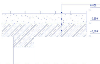
STROP GARÁŽE 1.PP
