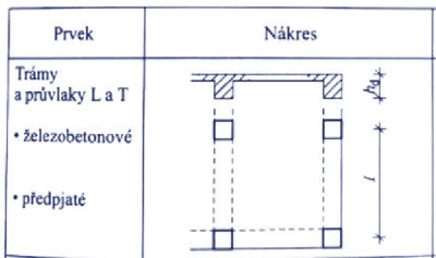
(obr. 2 – schéma železobetonový průvlak, str. 123 Navrhování nosných konstrukcí, doc. Ing. Karel Lorenz)
