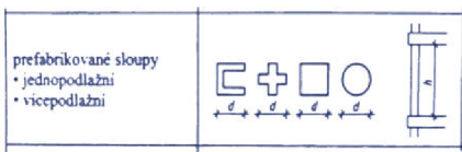
(obr. 3 – schéma prefabrikovaných ŽB sloupů, str. 174 Navrhování nosných konstrukcí, doc. Ing. Karel Lorenz)
