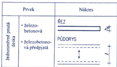
(obr. 1 – schéma jednosměrně pnuté desky železobetonové, str. 54 Navrhování nosných konstrukcí, doc. Ing. Karel Lorenz)
