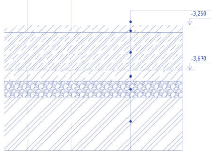
PODLAHA GARÁŽE 1.PP
