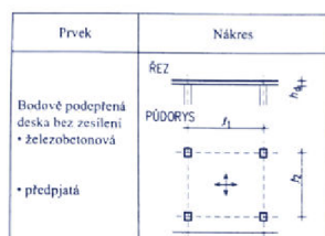
(obr. 4 – schéma bodově podepřené desky bez zesílení, str. 60 Navrhování nosných konstrukcí, doc. Ing. Karel Lorenz)
