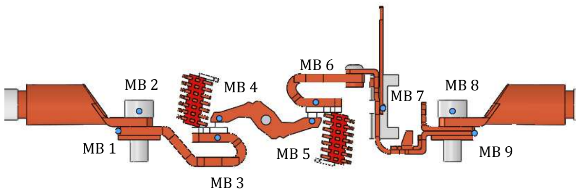
Obr. 4.3 Měřené body
