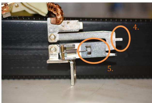
Obr. 3.2 Spoušť jističe s jedno kontaktním systémem
