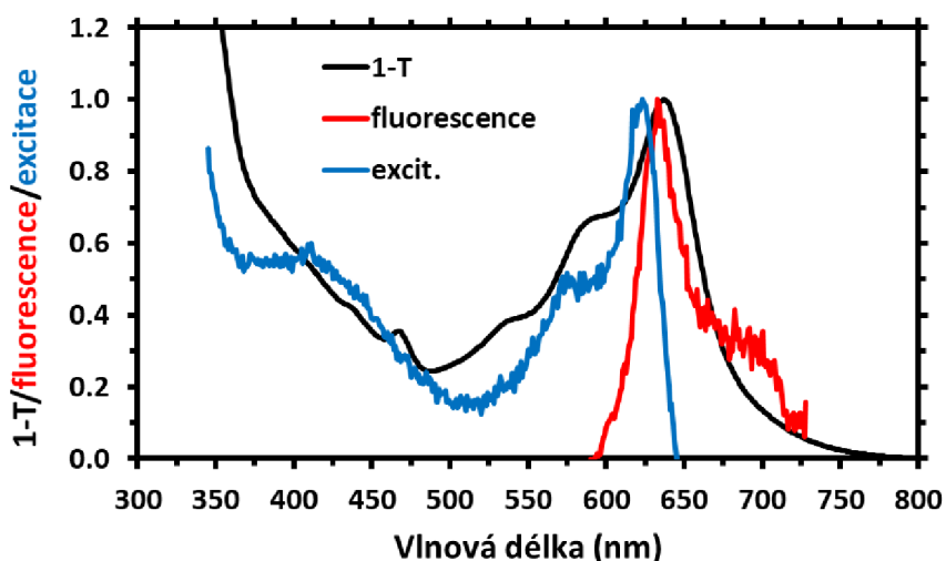
Obrázek 4.20: Emisní spektrum (červeně, excitace 580 nm), excitační spektrum (modře, detekce 680 nm) a 1-T (černě) pro fykocyanobilin s mědí v methanolu, jeden týden po přípravě vzorku. Spektra jsou normalizována na maximum signálu v oblasti
