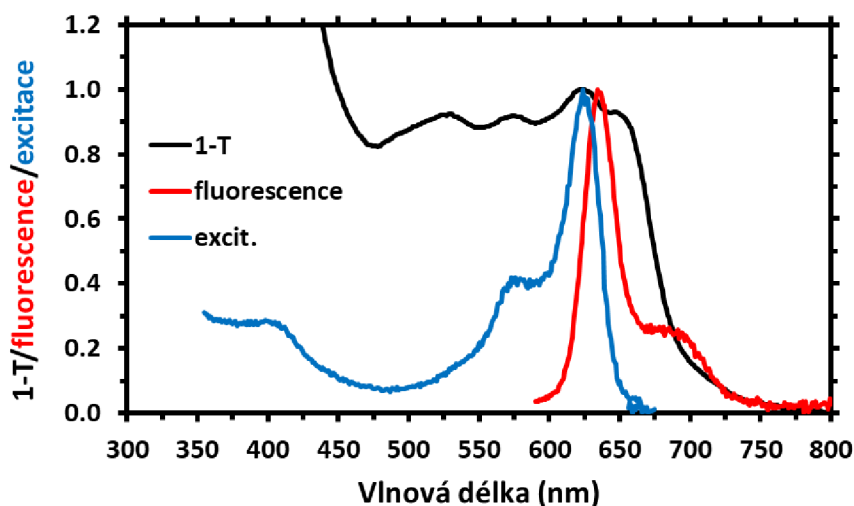
Obrázek 4.18: Emisní spektrum (červeně, excitace 580 nm), excitační spektrum (modře, detekce 680 nm) a 1-T (černě) pro fykocyanobilin s kobaltem v methanolu, jeden týden po přípravě vzorku. Spektra jsou normalizována na maximum signálu v oblasti Q pásu absorpčního spektra. Ramanův rozptyl methanolu by mohl být detekován u 698 nm.
