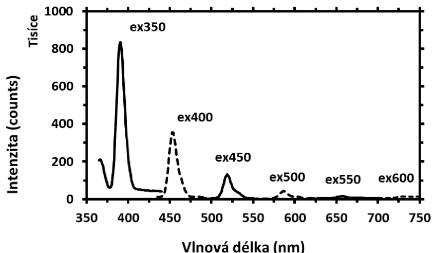
Obrázek 4.3: Ramanův rozptyl při různých excitacích vlnových délkách pro methanol.
