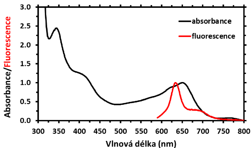
Obrázek 4.15: Absorpční spektrum (černě) a emisní spektrum (červeně) fykocyanobilinu s niklem v methanolu, jeden týden po přípravě vzorku (excitace 580 nm). Spektra jsou normalizována na maximum signálu v oblasti Q pásu absorpčního spektra. Ramanův rozptyl methanolu by mohl být detekován u 698 nm.
