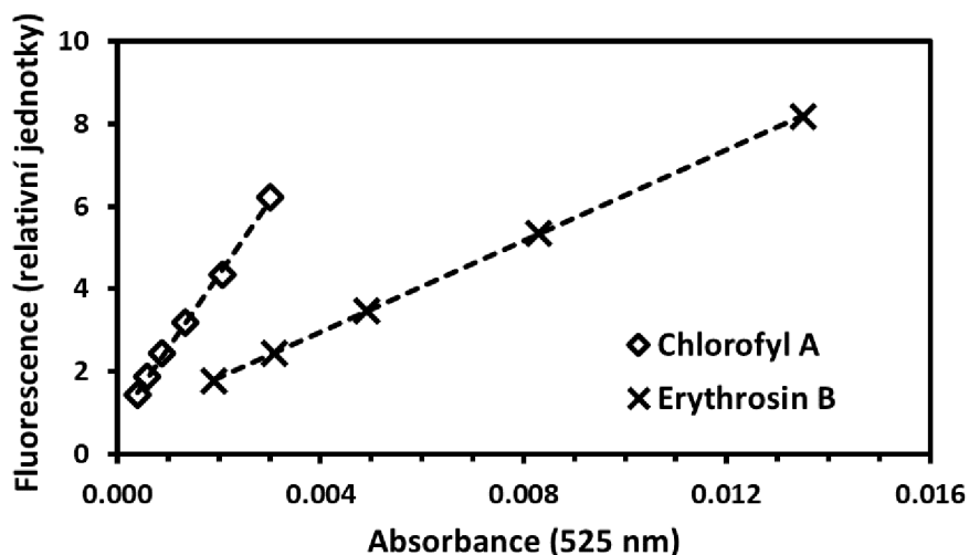
Obrázek 4.10: Graf závislosti integrované fluorescence na absorbanci koncentrační řady erythrosimu B a chlorofylu a k výpočtu kvantového výtěžku fluorescence chlorofylu a.
