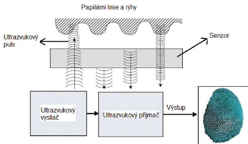
Obr. 4.2: Princip ultrazukové čtečky.
