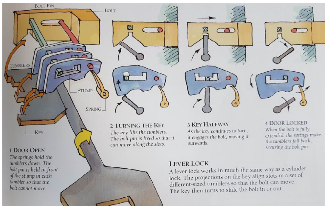
Obr. 1.2: Ukázka funkce západkového zámku.
