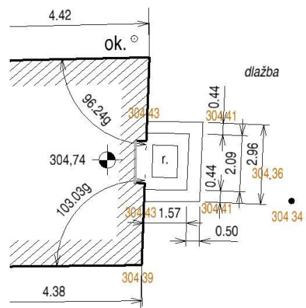
Obr. 122 Kóty schodů
