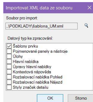
Obr. 30 Import XML souboru šablony prvků
