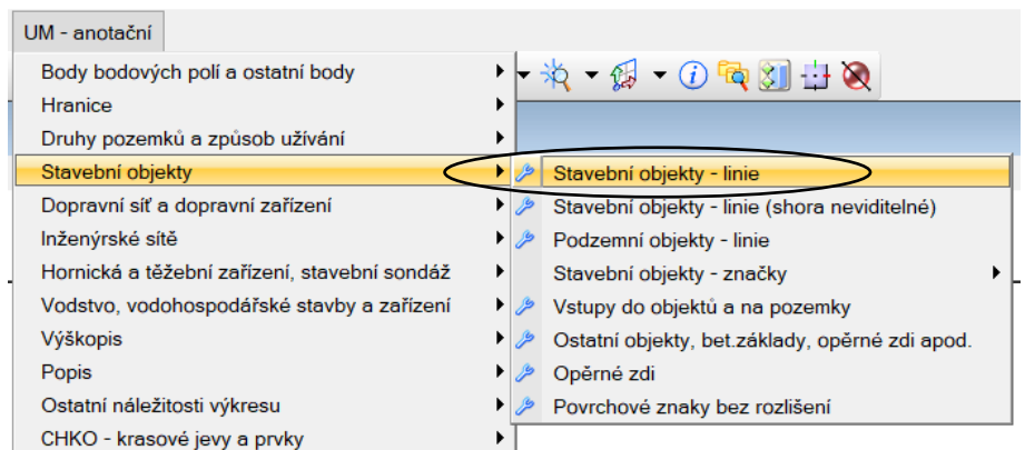
Obr. 90 Panel úloh pro stavební objekty – linie
