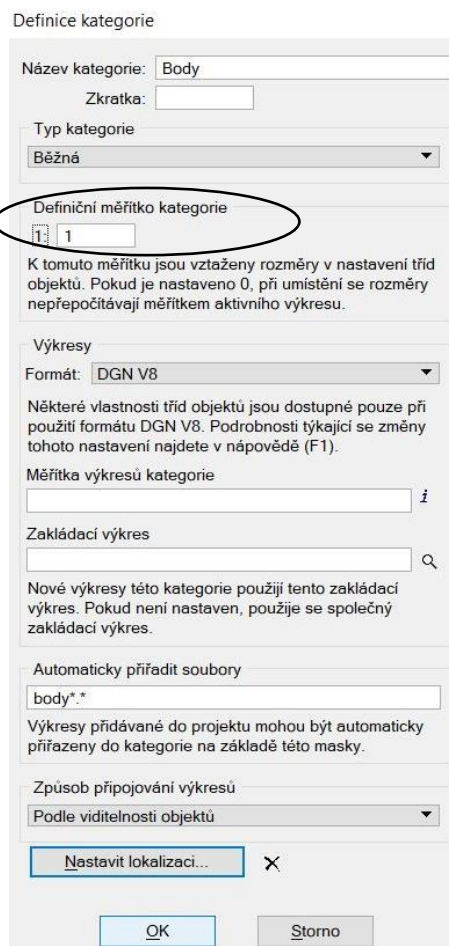
Obr. 84 Nastavení definičního měřítka kategorie Body
