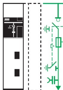
QM Skriňa s kombináciou odpínač-poistka 24 kV: 375 or 500 mm 36 kV: 750 mm
