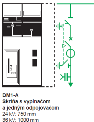
Obr. 7.2: Prívodné pole (Prevzaté z [25])
