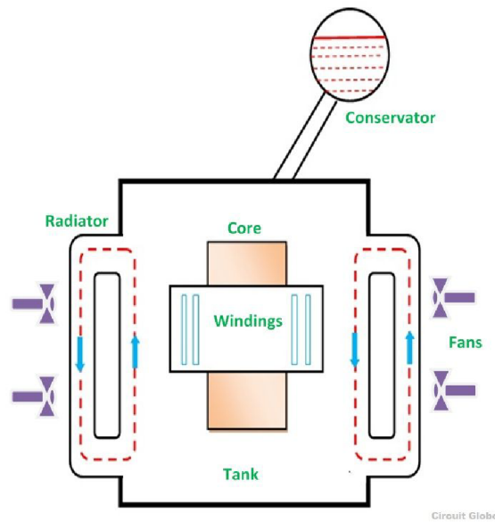
Obr. 1.2: ONAF chladienie (Prevzaté z [7])
