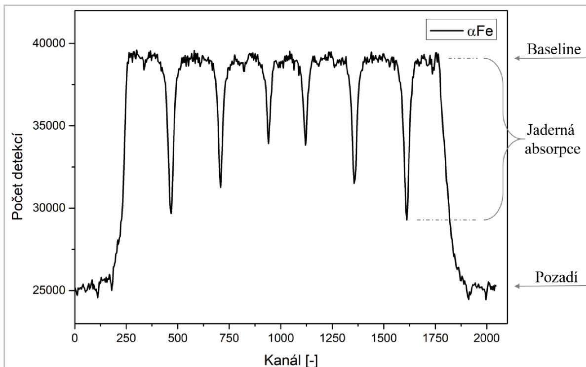
Obrázek 6: Rezonanční Mössbauerovské spektrum vzorku kalibračního železa o tloušťce 30 µm.
