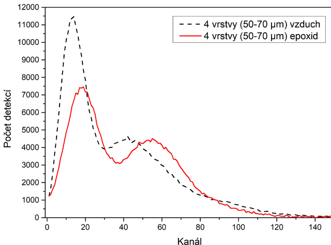
Obrázek 19: Amplitudová spektra 4 vrstev scintilátoru o zrnitosti 50-70 \mu\text{m} s mezerami vyplněnými vzduchem a epoxidovou pryskyřicí. Přebrato z [66], přeloženo.
