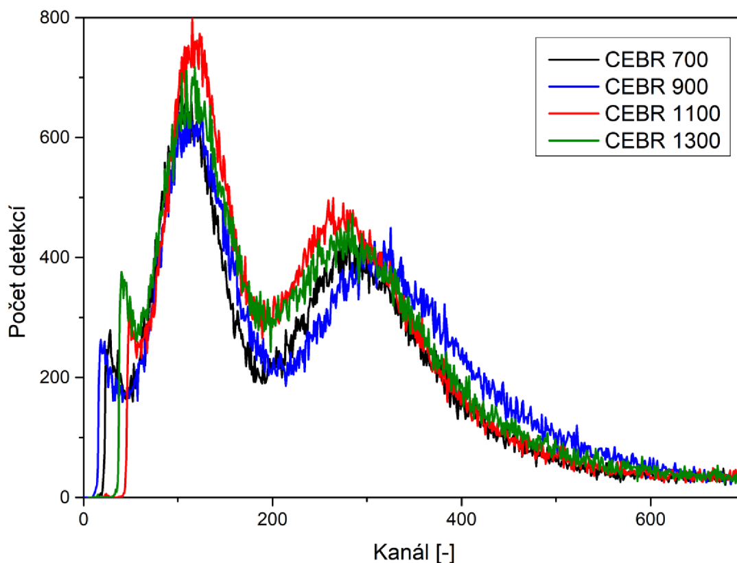
Obrázek 29: Amplitudová spektra scintilátorů CEBR 700 až CEBR 1300. Pro přehlednost je osa X jednotlivých spekter posunuta tak, aby se píky odpovídající energiím \langle 6,8 \rangle \text{ keV} překrývaly.
