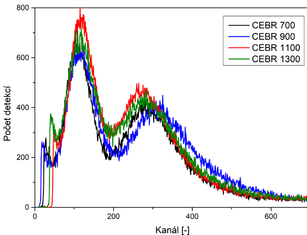
Obrázek 11: Amplitudová spektra scintilátorů CEBR 700 až CEBR 1300. Pro přehlednost je osa X jednotlivých spekter posunuta tak, aby se píky odpovídající energiím <6,8> keV překrývaly.
