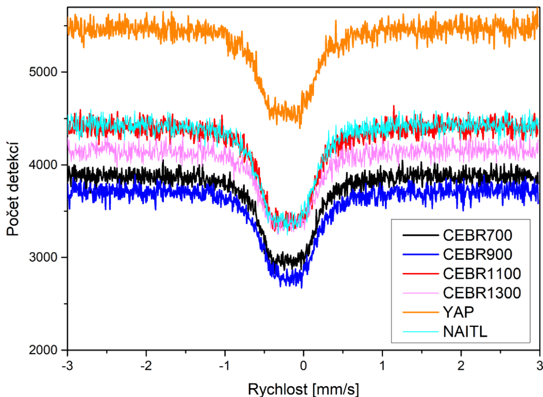
Obrázek 31: Mössbauerovská spektra vzorku FeAl měřená scintilátory CEBR700, CEBR900, CEBR1100, CEBR1300, NAITL a YAP.
