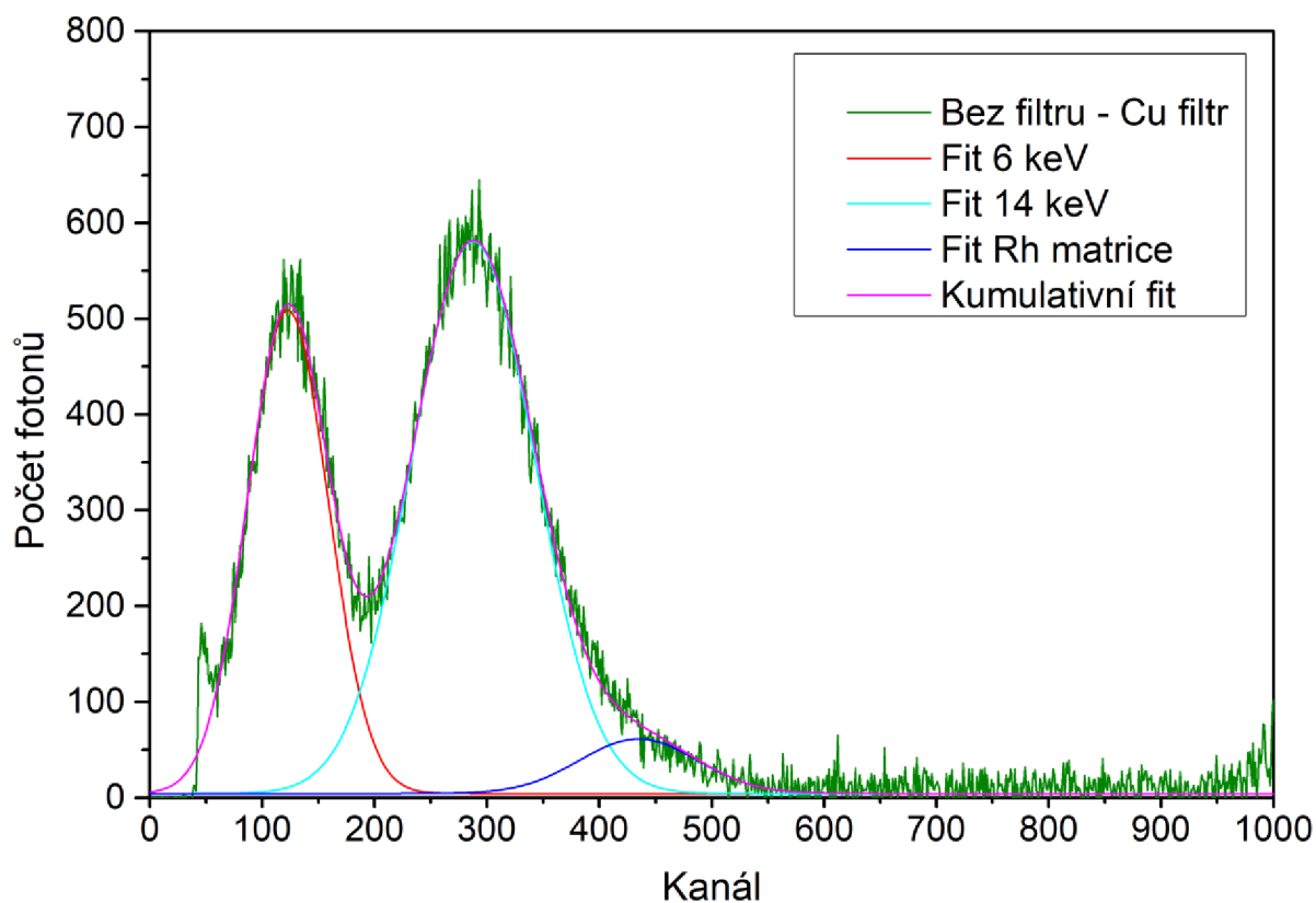
Obrázek 11: Amplitudové spektrum zářiče ^{57}\text{Co} zobrazené pomocí Gaussova rozdělení.
