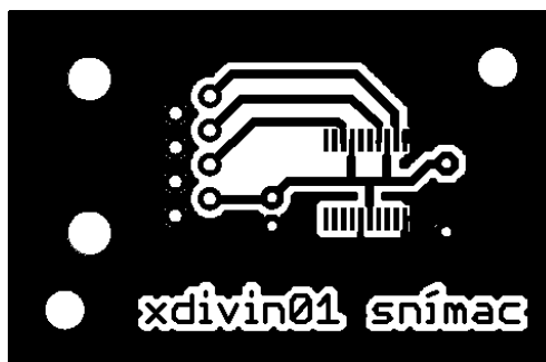
Obr. 3.6: Strana spojů plošného spoje snímače polohy točny.
