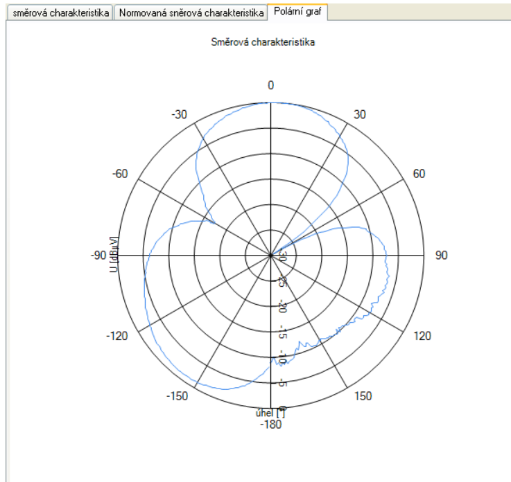
Obr. 6.3: Normovaná směrová charakteristika v polárním grafu.
