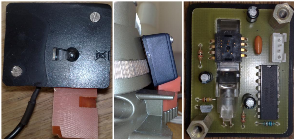
Obr. 3.2: Použitý snímač polohy.
