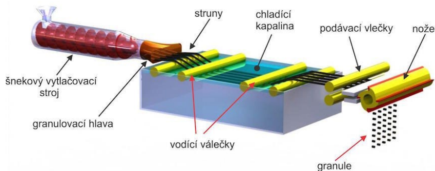
Obr.17 Granulace ze strun za studena [15o]
