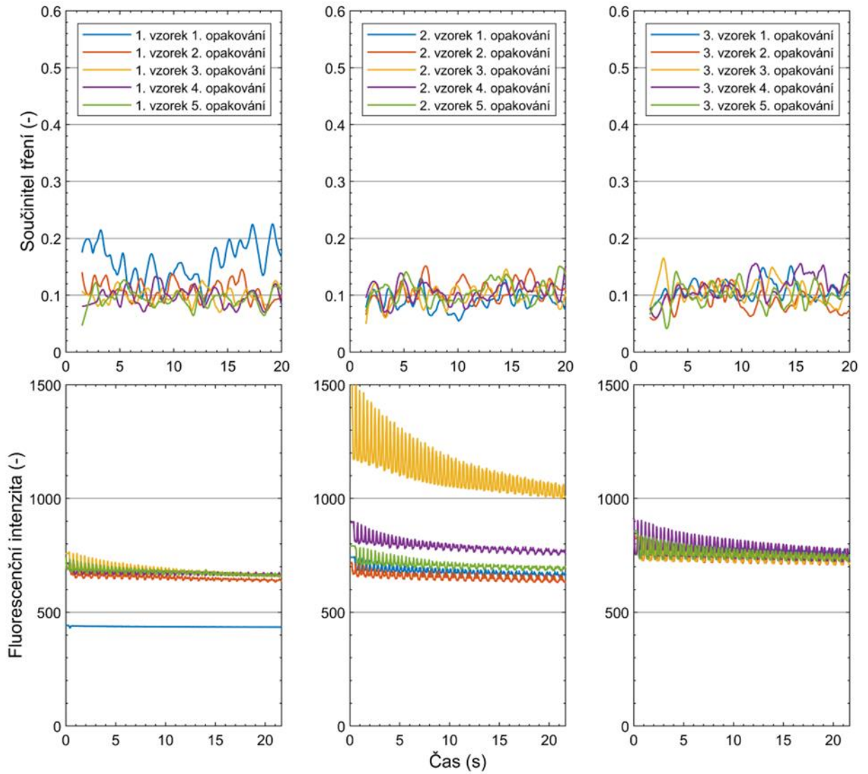
Obr. P2 – 7: Vývoj součinitele tření a fluorescenční intenzity v čase pro Acuvue Oasis HA337-HEPES
