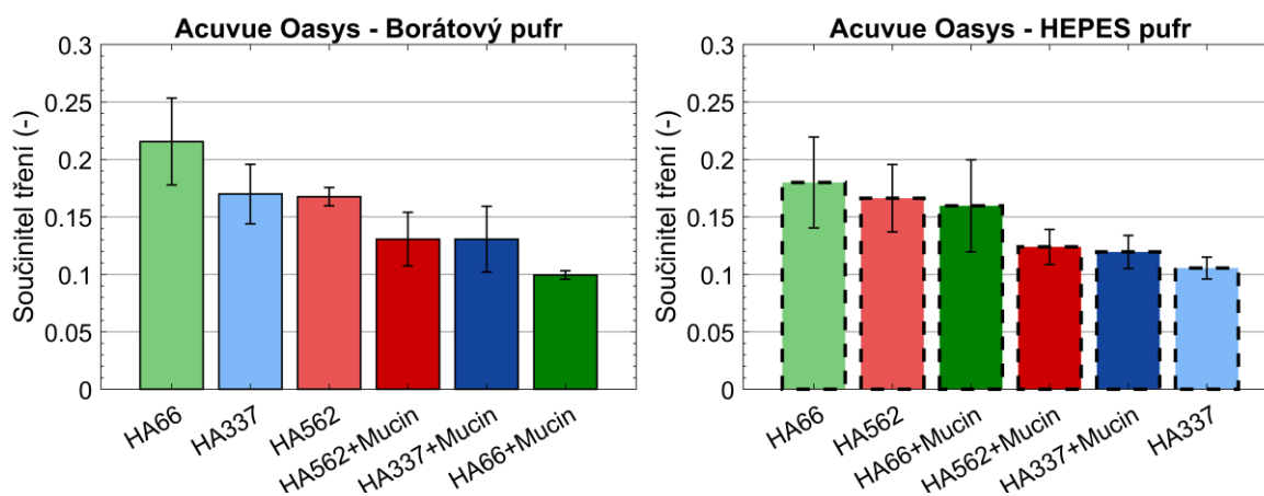
Obr. 5-3: Průměrný součinitel tŕení čoček Acuvue Oasys
