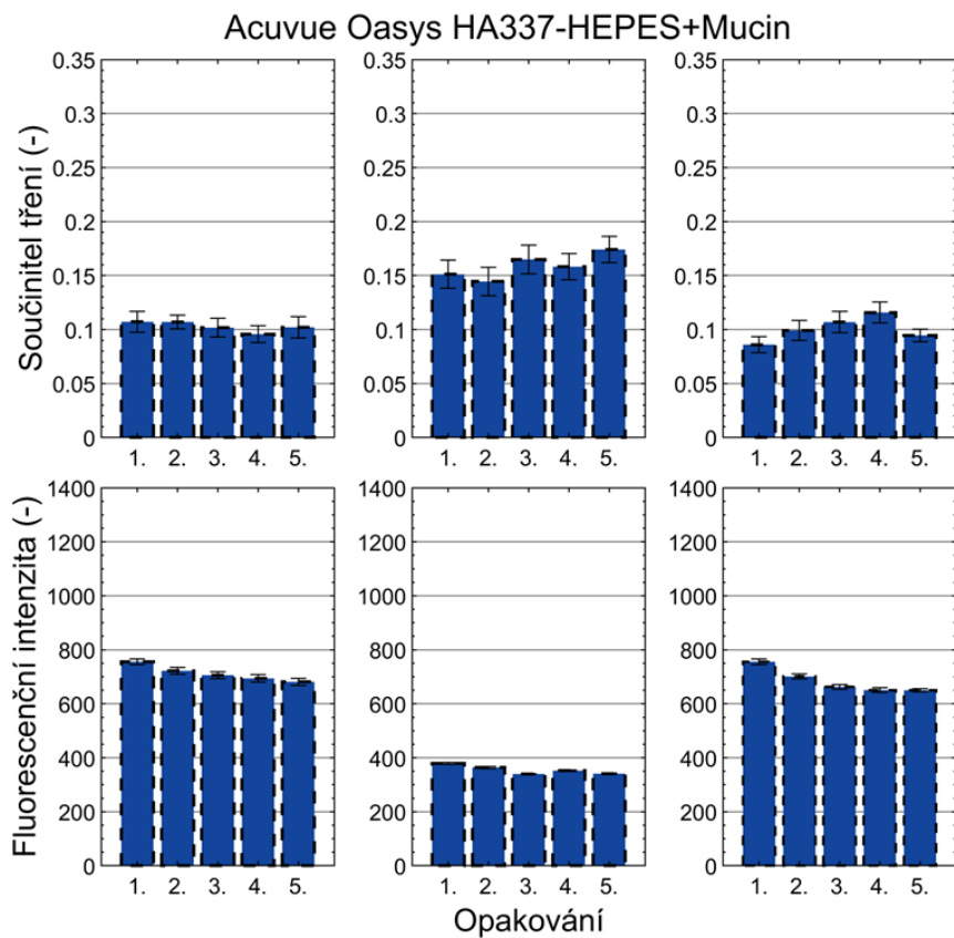
Obr. P1 – 8: Průměrný součinitel tření a fluorescenční intenzity opakovaných měření Acuvue Oasys HA337-HEPES+Mucin
