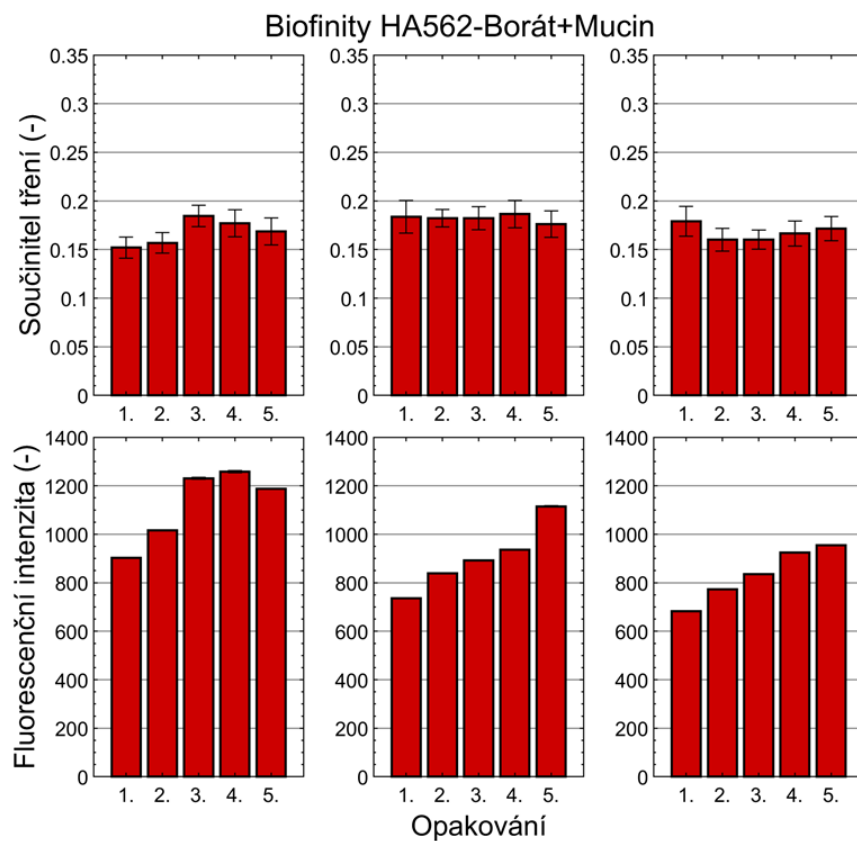
Obr. P1 – 22: Průměrný součinitel tření a fluorescenční intenzity opakovaných měření Biofinity HA562-Borát+Mucin
