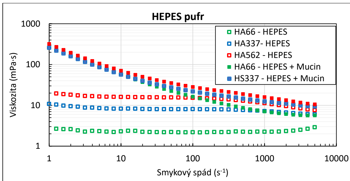
Obr. 5-2: Tokové křivky roztoku KH v HEPES-pufu
