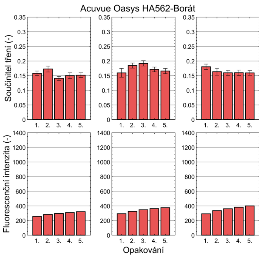
Obr. P1 – 9: Průměrný součinitel tření a fluorescenční intenzity opakovaných měření Acuvue Oasys HA562-Borát
