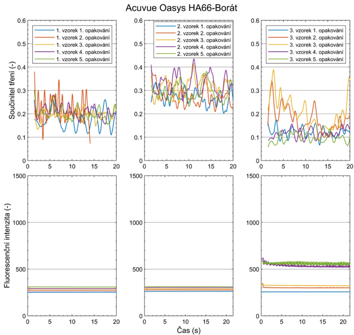
Obr. P2 – 1: Vývoj součinitele tření a fluorescenční intenzity v čase pro Acuvue Oasys HA66-Borát
