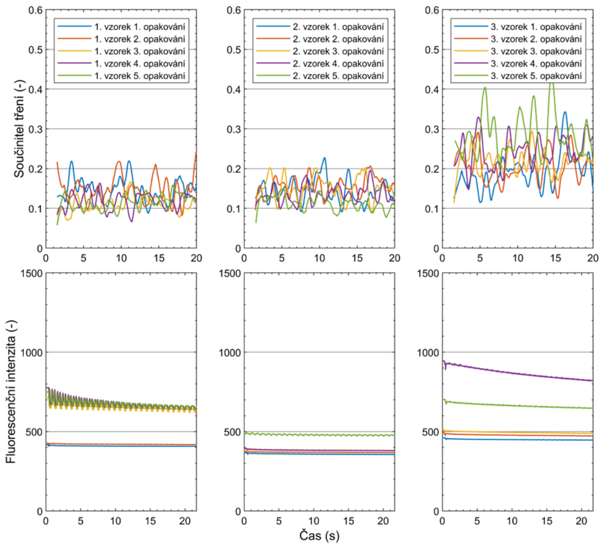
Obr. P2 – 11: Vývoj součinitele tření a fluorescenční intenzity v čase pro Acuvue Oasys HA562-HEPES
