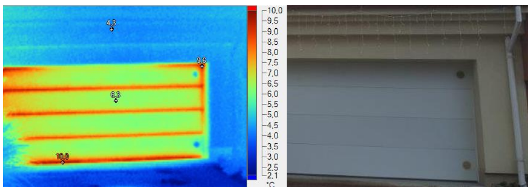
Obr. 35 Garážová vrata
