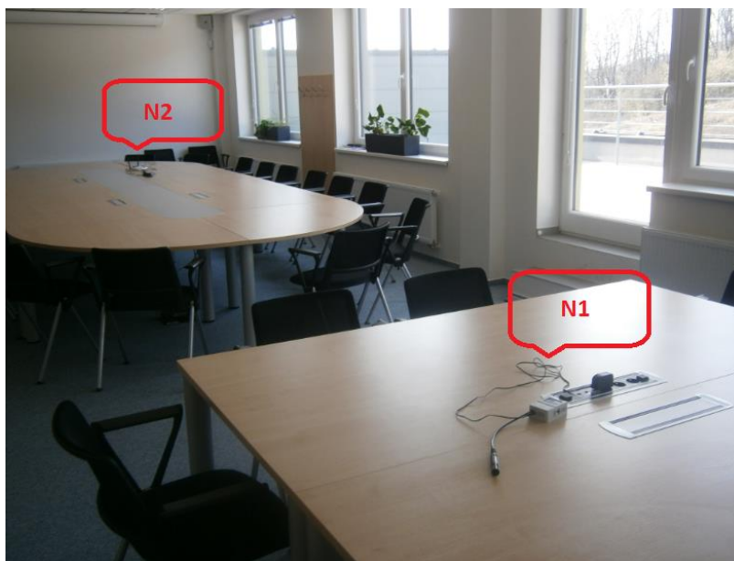
Obr. 50 Poloha měřidel v zasedací místnosti
