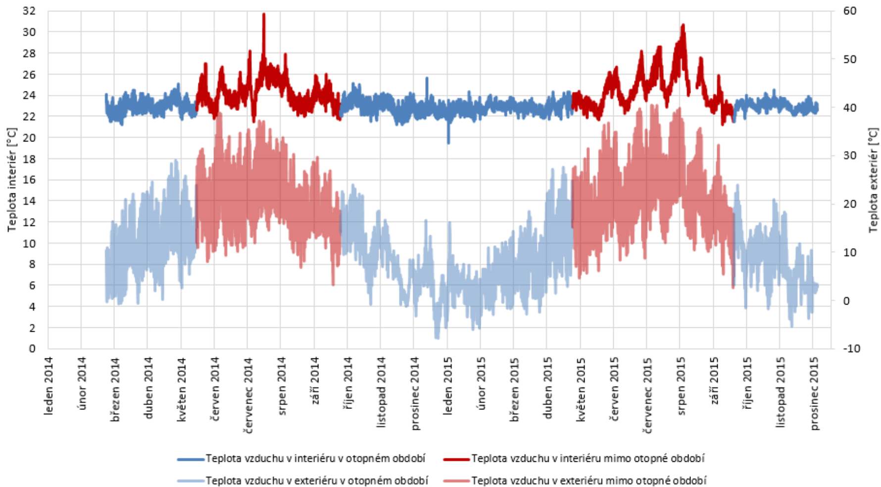
Graf 11 - Průběh naměřené teploty vzduchu v interiéru a exteriéru
