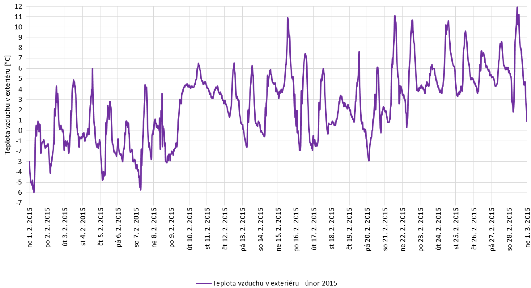
P2 - Průběh teploty vzduchu v exteriéru v měsíci únor 2015
