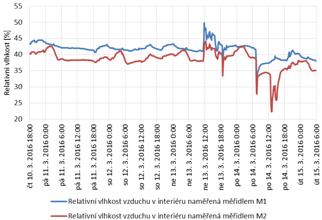
Graf 2 - Průběh relativní vlhkosti vzduchu v obývacím pokoji
