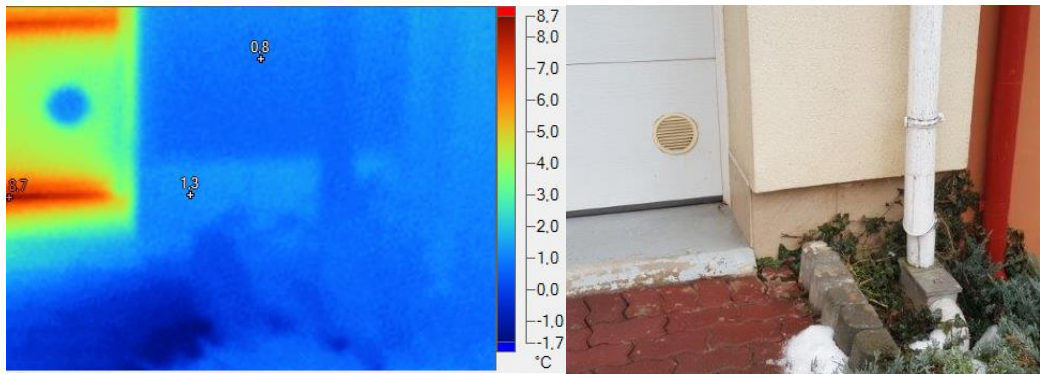
Obr. 36 Sokl
