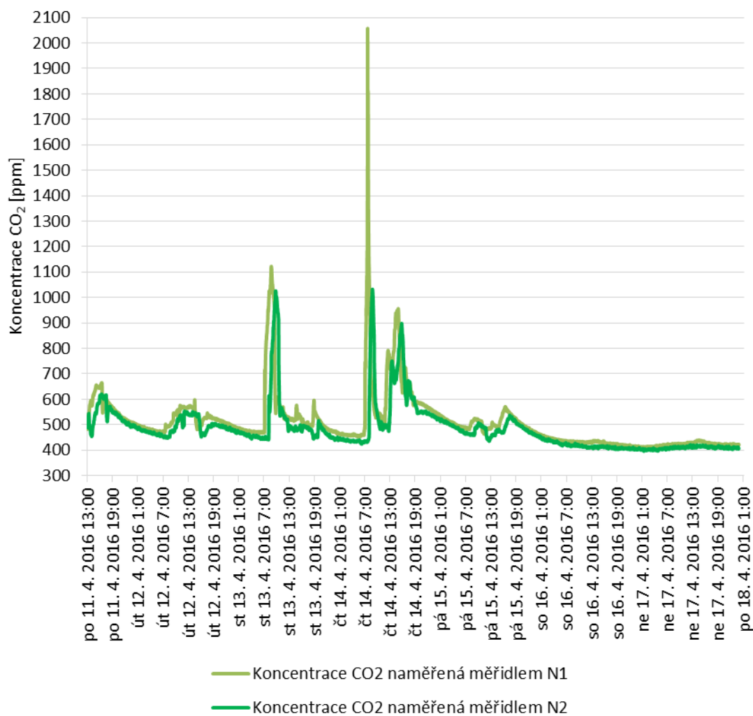
Graf 9 - Průběh naměřené koncentrace CO 2 měřidlem N1 a N2
