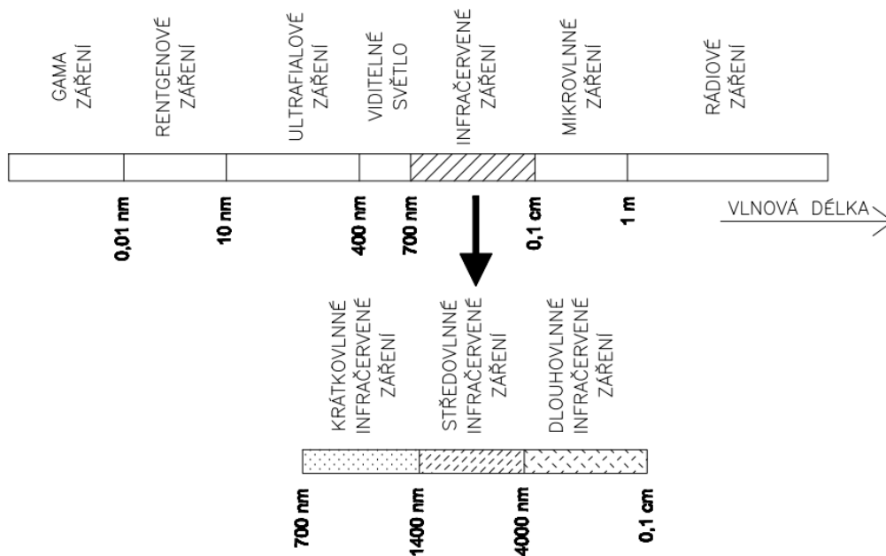
Obr. 4 Elektromagnetické spektrum
