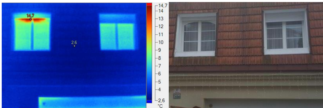
Obr. 34 Pohled na obvodový plášť z ulice
