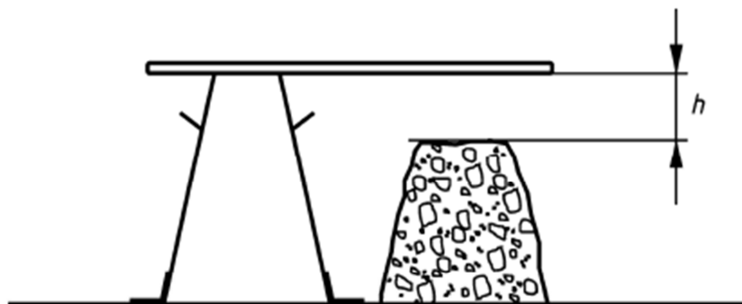
Obrázek 1 – Měření sednutí
