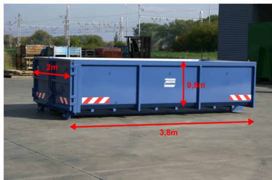
[3.7]: Kontejner 6 m 3 / 3 t
