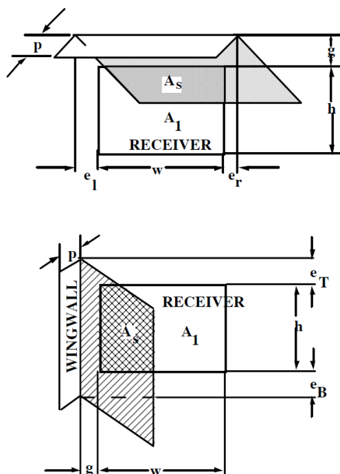
Obr. 5.12: Geometrie stínění [35].
