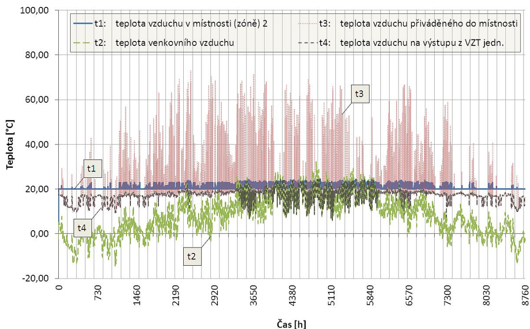
Obr. 5.21: Var. A2 - průběh teplot během celého roku (chování iVZT systému)
