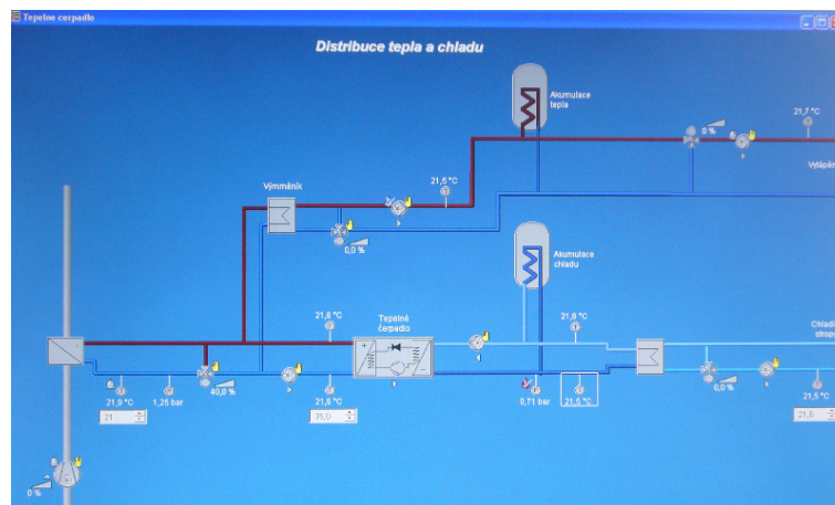
Obr. B.5: Nastavení zdroje chladu v počítači.
