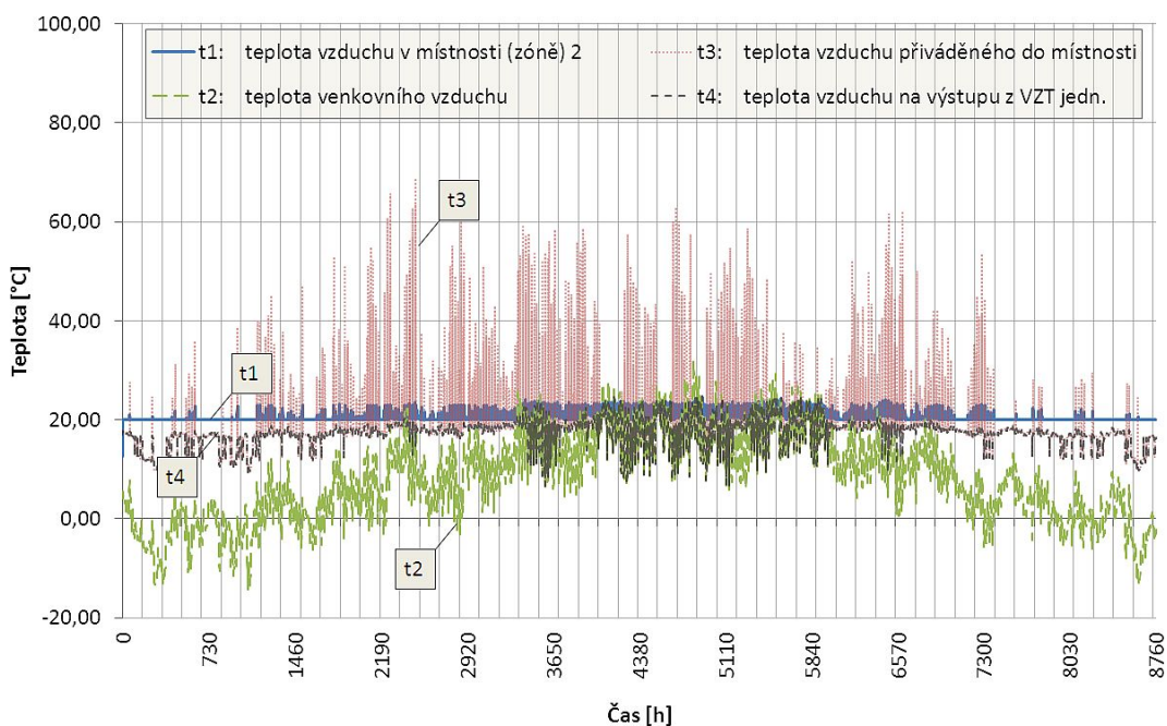
Obr. 5.19: Var. A1 - průběh teplot během celého roku (chování iVZT systému)
