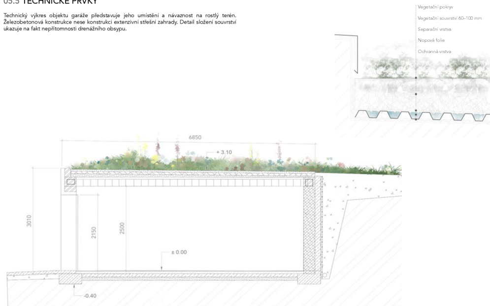
obr. 67 Technický prvek – garáž obr. 68 Detail souvrství
