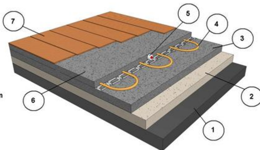
Obrázek 3: Podlahové topení [19]
