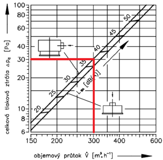
Obrázek 2.11 Tlaková ztráta a akustický výkon VVM 500/16
