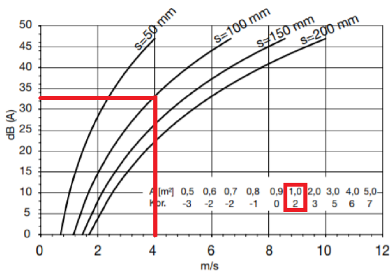
Obrázek 2.33 Hladina hluku tlumiče na přívodu exteriér
