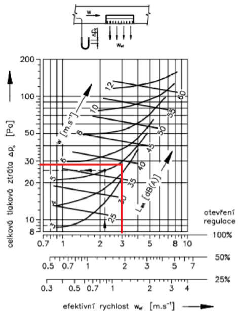
Obrázek 2.22 Tlaková ztráta, akustický výkon a rychlost proudění VNKM 1225x225
