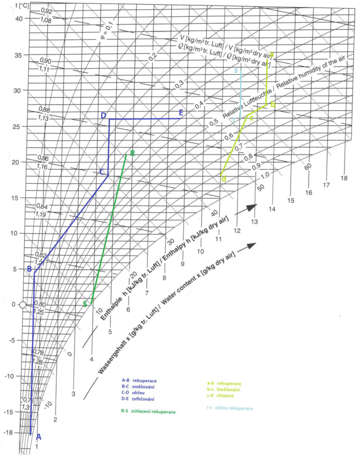
Obrázek 2.26 H-x diagram zařízení č. 2
