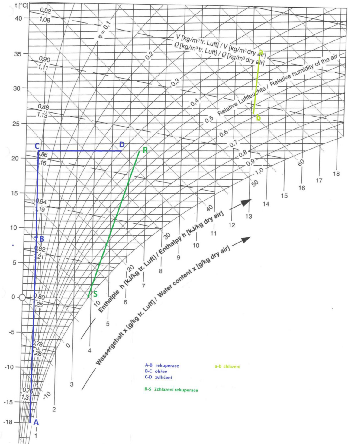
Obrázek 2.25 H-x diagram zařízení č. 1
