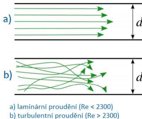
Obrázek 1.7 Typy proudění vzduchu v potrubí
