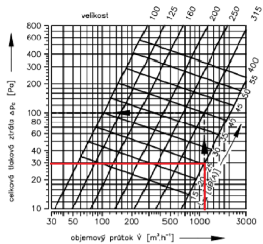
Obrázek 2.19 Tlaková ztráta a akustický výkon DDM II 400/S
