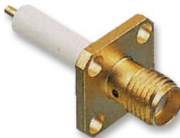
Obrázek 4.1: Vzhled konektoru RADIALL R12541400 RF.
