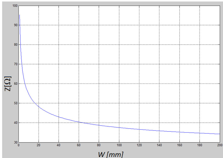
Obrázek 2.4: Závislost impedance na šířce středního vodiče.
