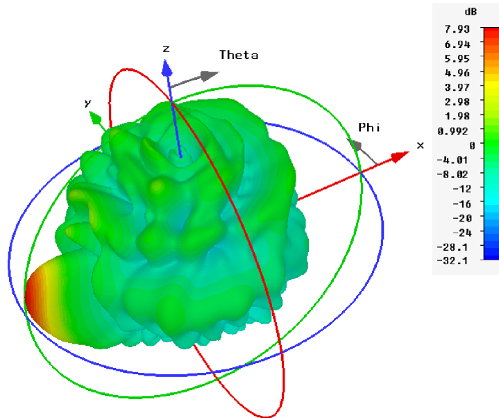
Obrázek 5.27: 3D vyzařovací charakteristika směrové antény s prstem umístěným na pinu konektoru.
