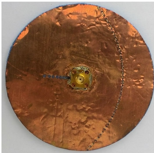
Obrázek 6.6: Vyrobená směrová monopólová anténa ze strany konektoru.
