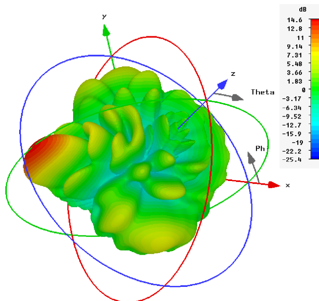
Obrázek 4.14: 3D vyzařovací charakteristika směrové monopólové antény s parabolou a s direktory.
