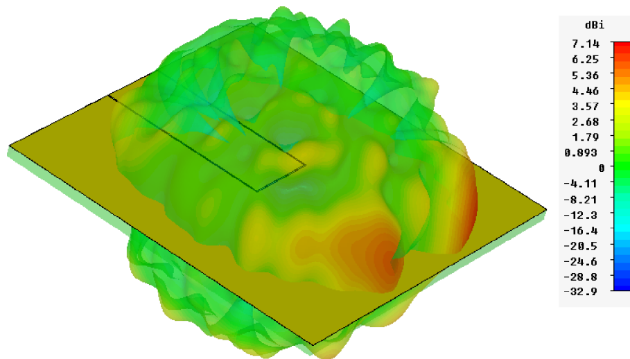
Obrázek 2.6: Vyzařovací 3D charakteristika koplanárního vlnovodu.
