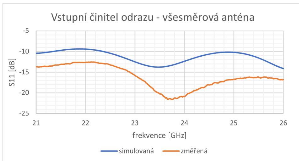
Obrázek 6.3: Graf vstupního činitele odrazu vyrobené a simulované všesměrové monopólové antény.
