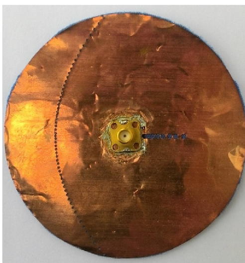
Obrázek 6.1: Vyrobena všesměrová monopólová anténa ze strany konektoru.
