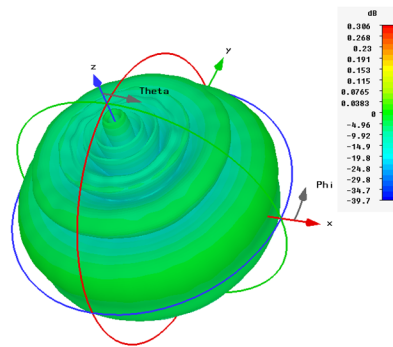
Obrázek 5.1: 3D vyzařovací charakteristika všesměrové antény s deskou vyrobené z PET ve vzdálenosti 0 mm.
