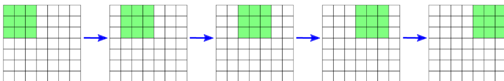
Obrázek 4.6: Posuv filtrového okna s krokem 1. Výstupní obrázek bude o rozměrech 5 \times 5 .
