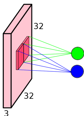
Obrázek 4.4: Neurony první vrstvy neuronové sítě namapované na lokální receptivní pole.
